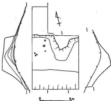
第6図 第1-a区空堀実測図
