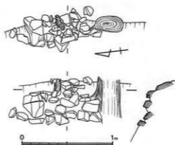
第10図 石垣遺構実測図
