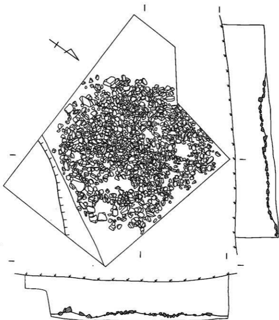
第8図 石積遺構実測図(第2-d区)
