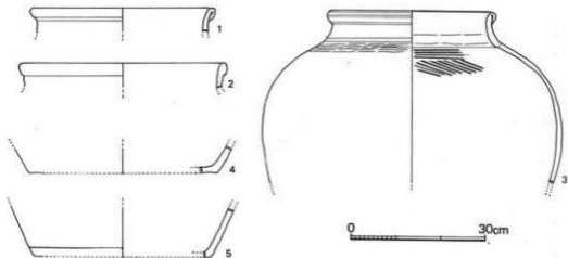
第11図 陶器実測図
