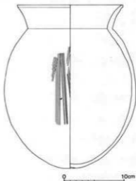
第2図 土師器実測図
