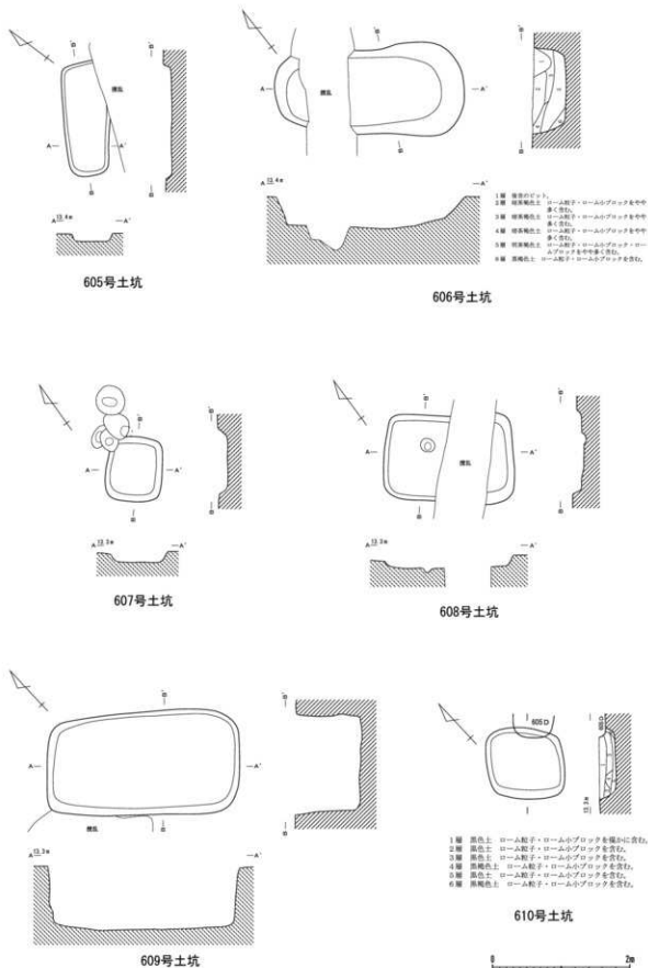
第42図 土坑 (1/60)
