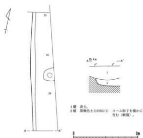
第17図 5号溝跡 (1/60)
