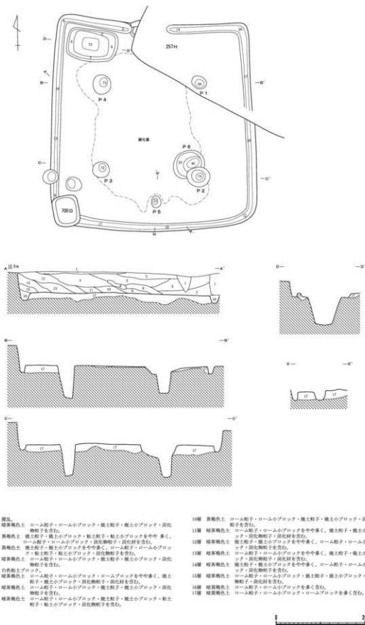
第12図 256号住居跡 (1/60)
