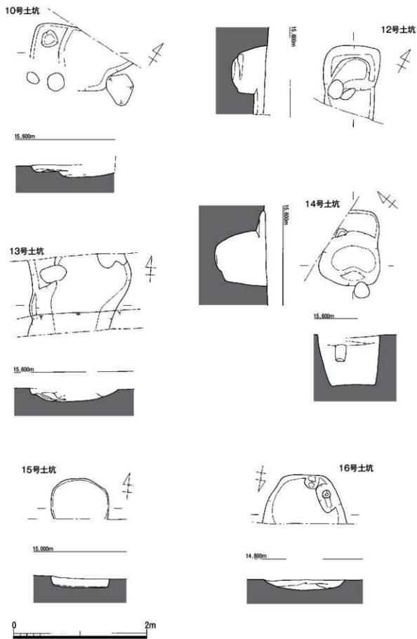
第8图 B区 土坑实测图② (S=1/40)
