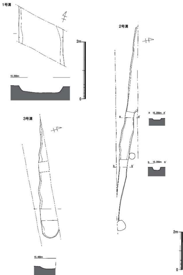
第10図 B区 溝実測図① (1号溝は S=1/40 、2・3号溝は S=1/60 )
