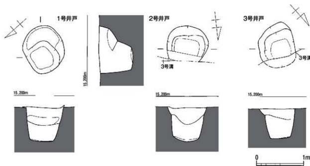
第9図 B区 井戸実測図 (S=1/40)
