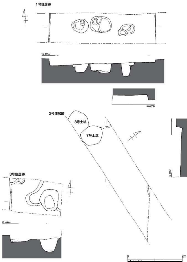
第6图 B区 住居跡实测图 (S=1/40)
