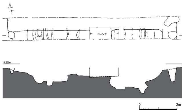
第13図 B区 流路跡実測図 (S=1/60)
