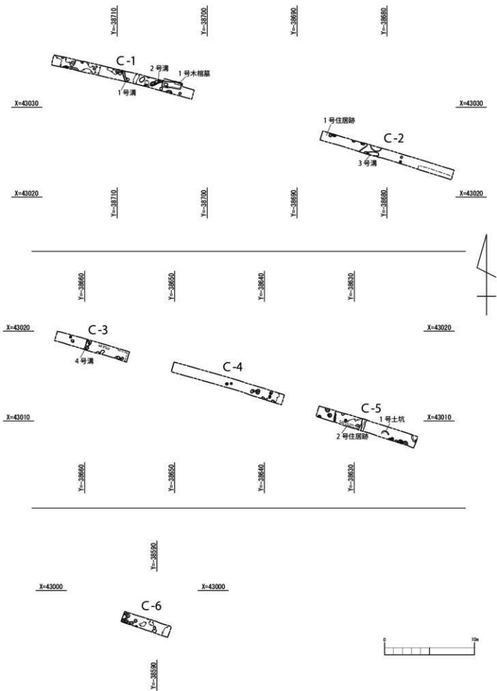
第15图 C区 遺構全体图 (S=1/300)
