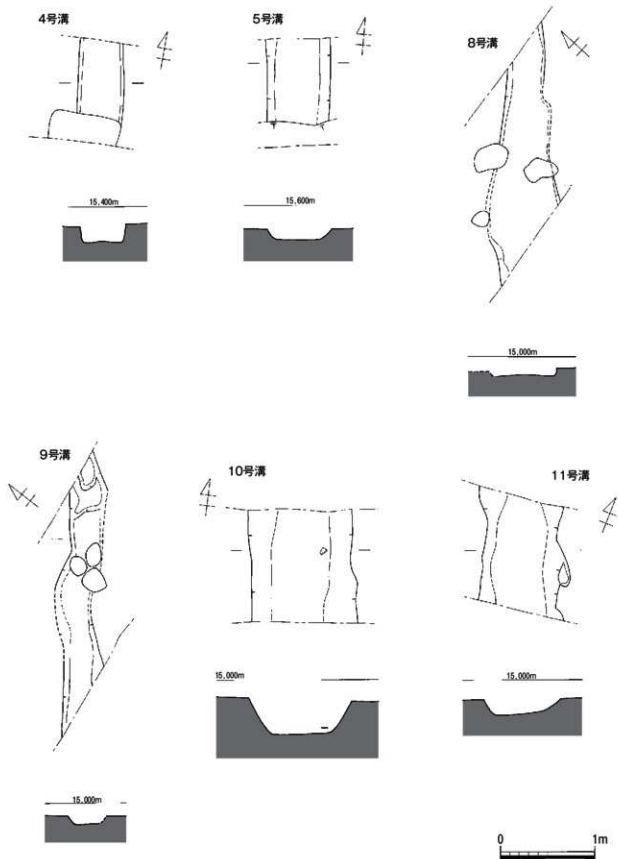
第11图 B区 沟实测图② (S=1/40)
