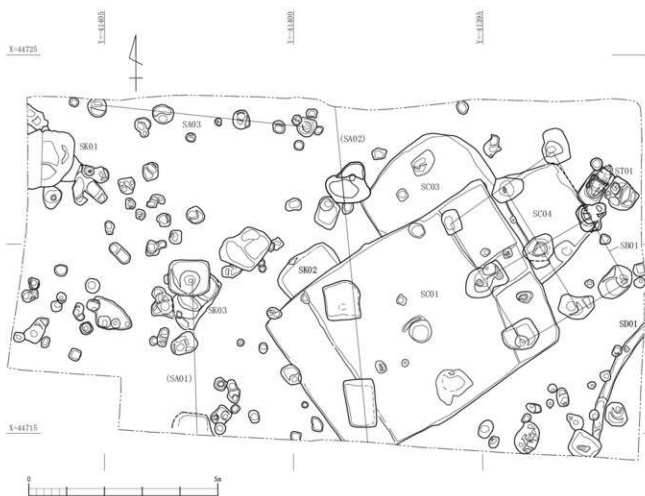
第2図 小郡若山遺跡9全体図 (s = 1/100)
