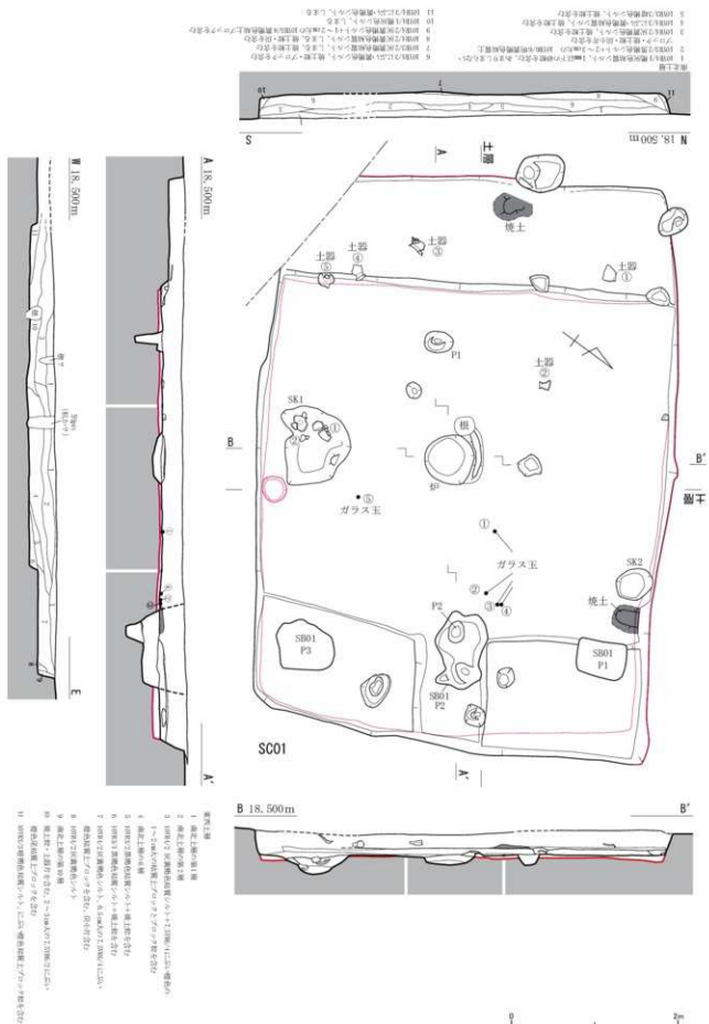
第3図 1号住居跡 実測図 (s = 1/50)
