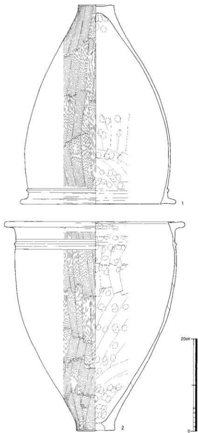
第13图 1号瓷棺 实测图 (s = 1/4)
