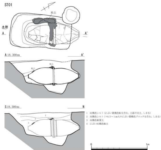
第12図 1号甕棺墓 実測図 (s = 1/20)
