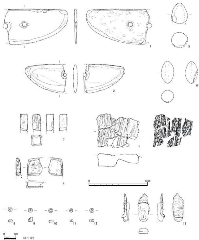
第14図 小郡若山遺跡9出土石器・土製品・ガラス製品・鉄器実測図 (s = 1/1, 1/2)
