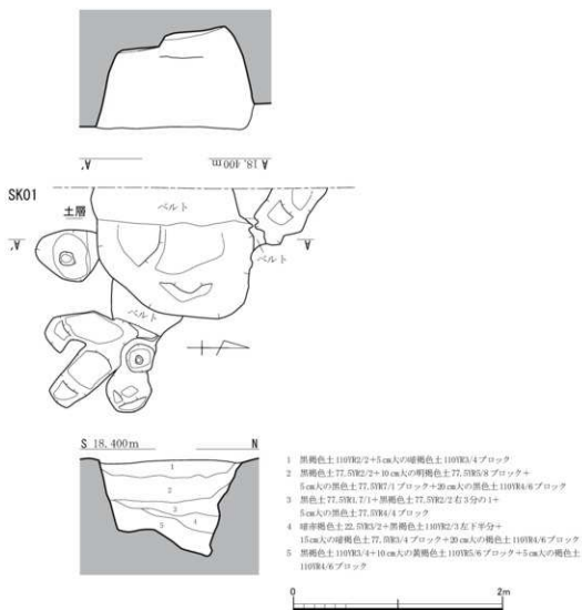
第17図 1号土坑 実測図 (s = 1/40)
