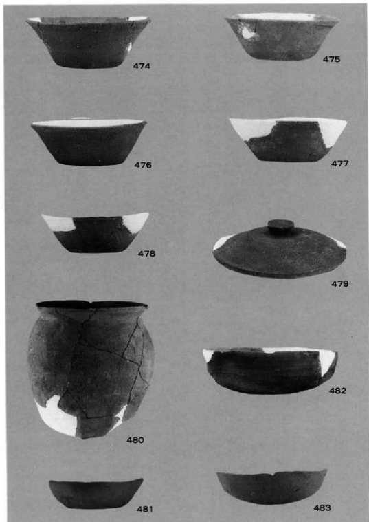
第118・120号住居跡出土遺物，474～480(SI-118)，481～483(SI-120)
