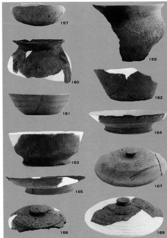
第44・45号住居跡出土遺物, 157~160(SI-44), 161~169(SI-45)
