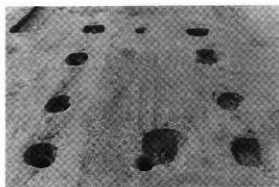
第 5 号掘立柱建物跡
