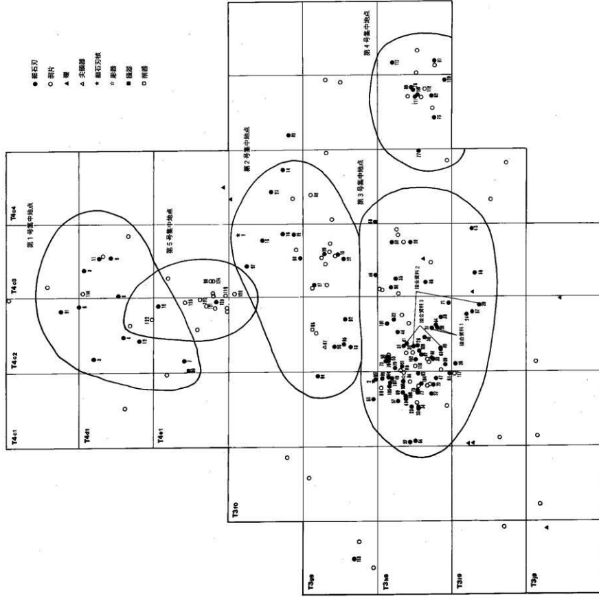
第31图 器種別石器集中地点平面图
