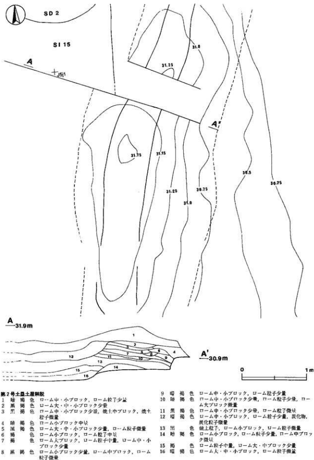
第49図 第2号土塁実測図
