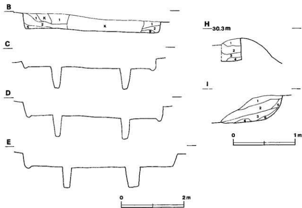
第36图 第19号住居跡実測図
