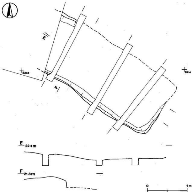
第9図 第1主体部掘り方
