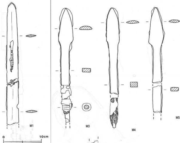
第13图 第1主体部 出土遺物実測図
