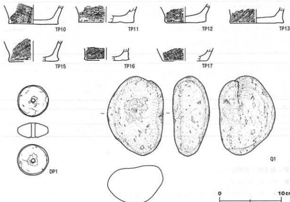
第19図 第1号住居跡出土遺物実測図(2)
