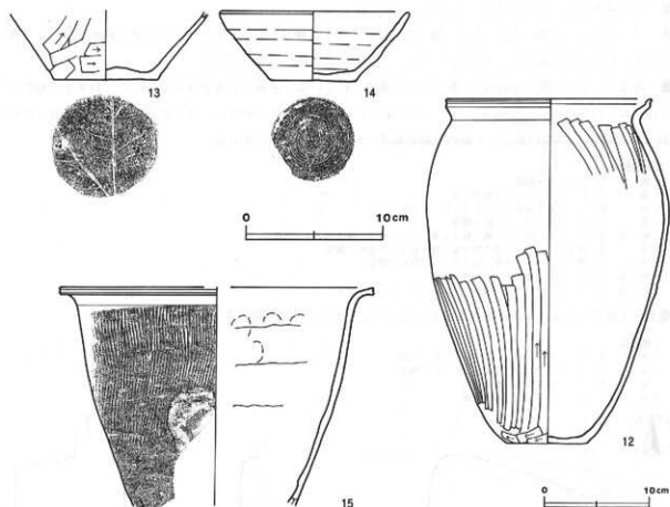
第23図 第3号住居跡出土遺物実測図
