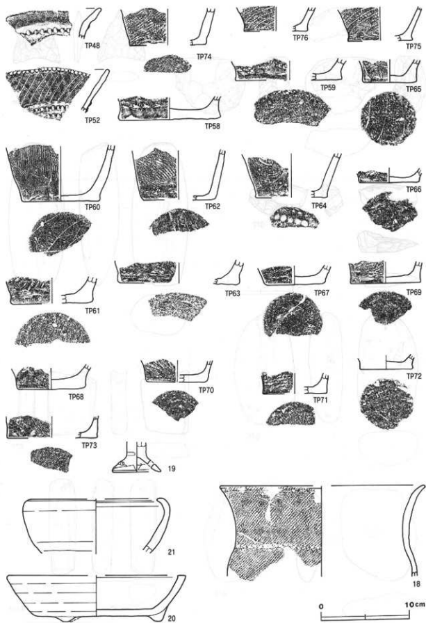
第29图 遺構外出土遺物実測図(3)
