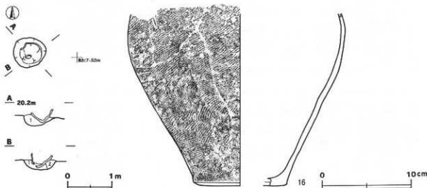
第20図 第1号土坑・出土遺物実測図
