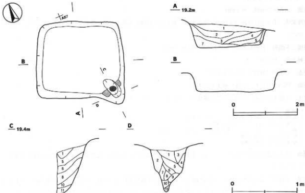
第24図 第4号住居跡実測図
