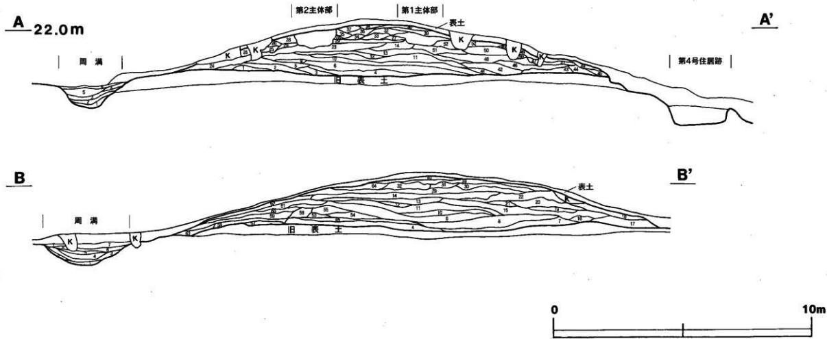
第7図 愛宕山古墳横丘・周溝土層図
