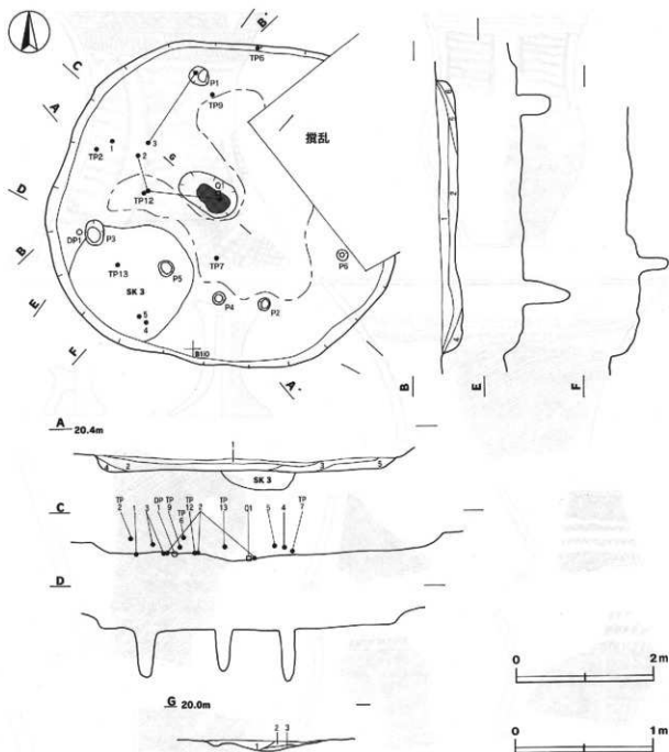
第17図 第1号住居跡実測図
