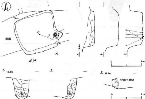
第22図 第3号住居跡実測図
