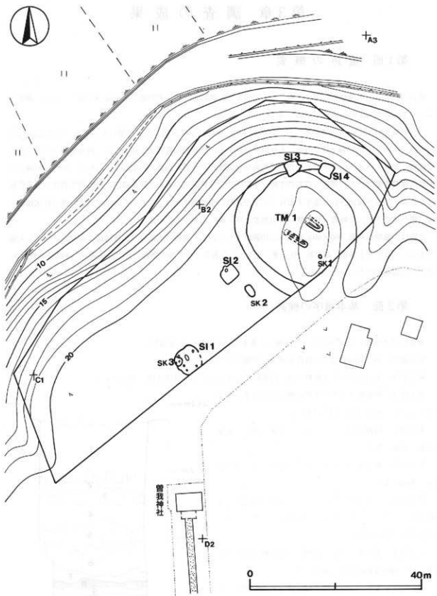
第4図 愛宕山古墳遺構全体図
