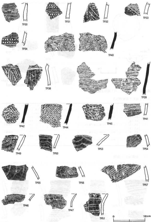
第28図 遺構外出土遺物実測図(2)
