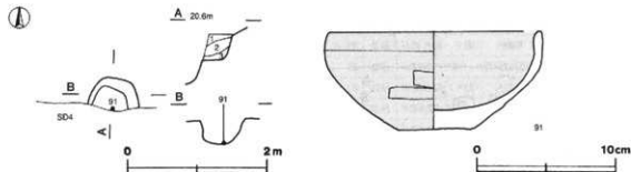
第16図 第80号土坑・出土遺物実測図
