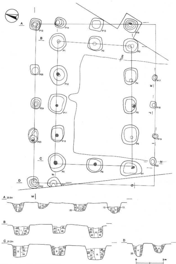
第22图 第1号插立柱建物跡実測図
