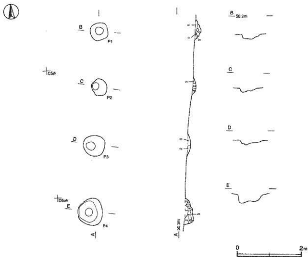
第171図 第14号柵跡実測図
