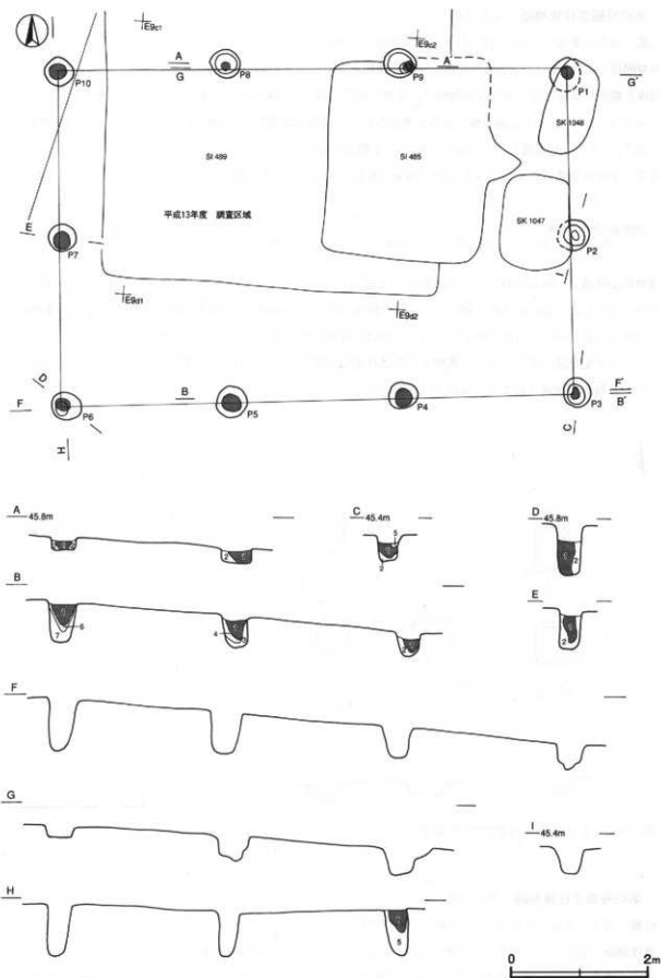
第132图 第12号掘立柱建物跡実測图
