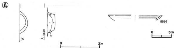
第146図 第1717号土坑・出土遺物実測図
