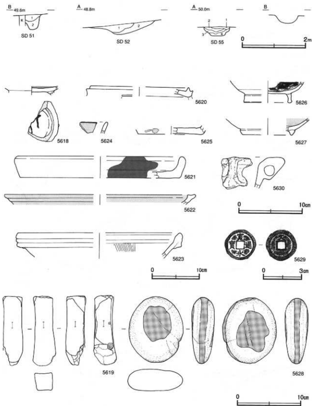
第169图 第51·52·55号沟迹土层断面图，第38·42·44·45·52号沟迹出土物实测图
