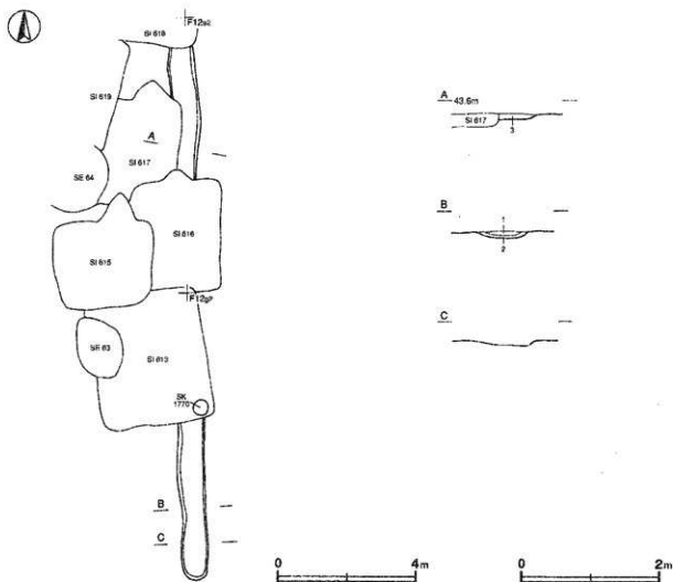
第143図 第37号清跡実測図
