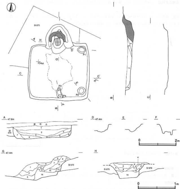
第129図 第669号住居跡実測図
