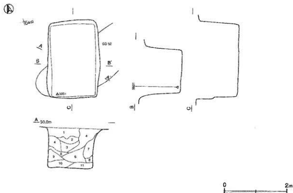
第158図 第2045号土坑実測図
