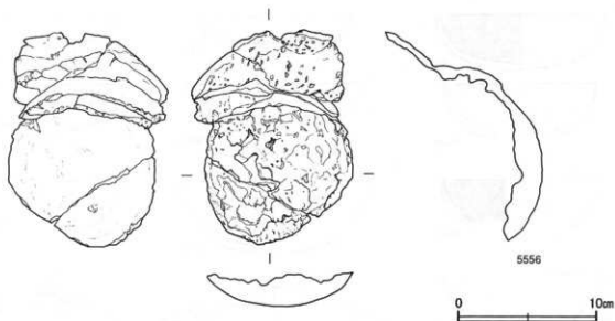
第139図 第2号鍛冶工房跡出土遺物実測図(2)
