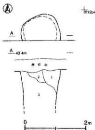
第165図 第66号井戸跡実測図
