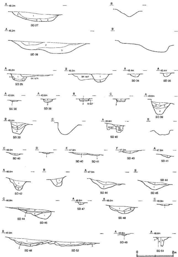
第168图 第27~29·34~36·38~42·44·45·47~49·51·52号沟迹上树断面图
