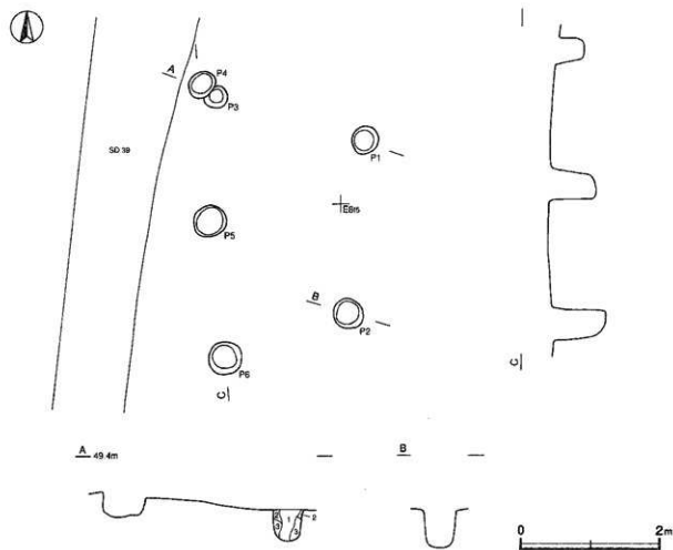
第174図 第41号ビット群実測図
