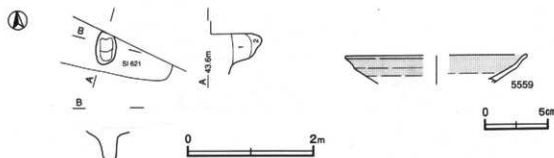
第144図 第1646号土坑・出土遺物実測図
