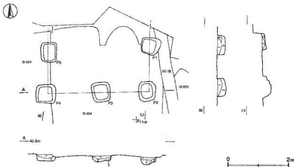
第133図 第42号掘立柱建物跡実測図
