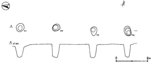
第173図 第16号横跡実測図
