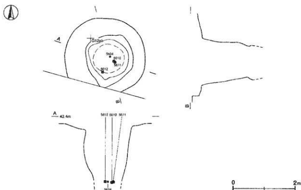
第141図 第60号井戸跡実測図
