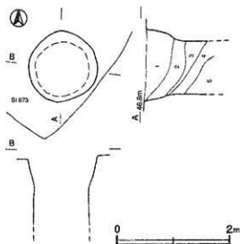
第167図 第68号井戸跡実測図
