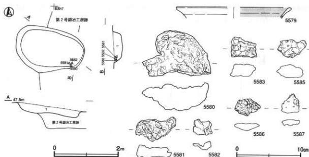
第152図 第1877号土坑・出土遺物実測図
