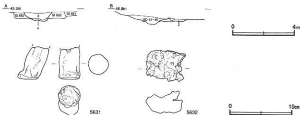
第170図 第1号道路跡土層断面・出土物実測図
