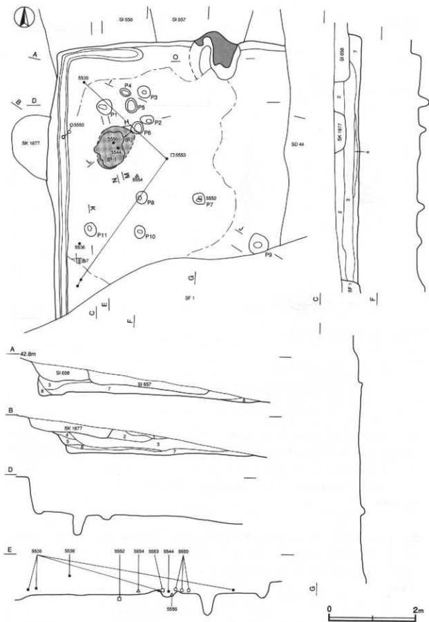
第135图 第2号锻冶工房跡实测图(1)
