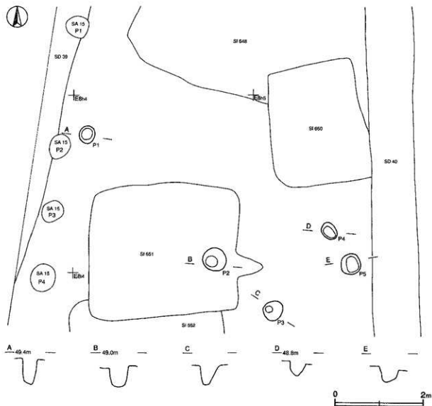
第175図 第42号ピット群実測図
