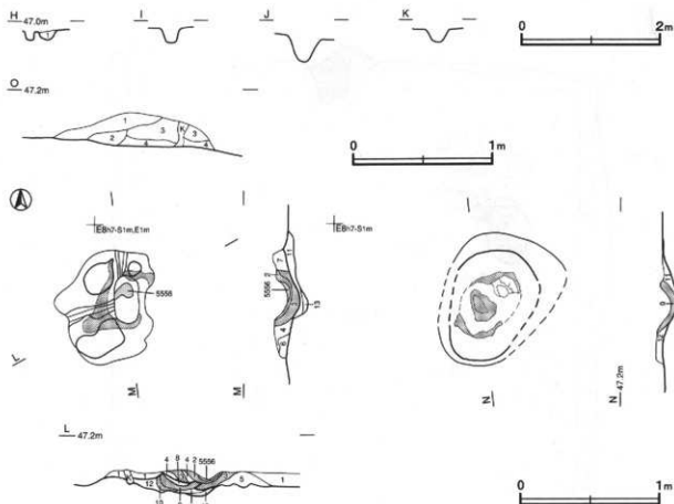
第136図 第2号鍛冶工房跡実測図(2)
