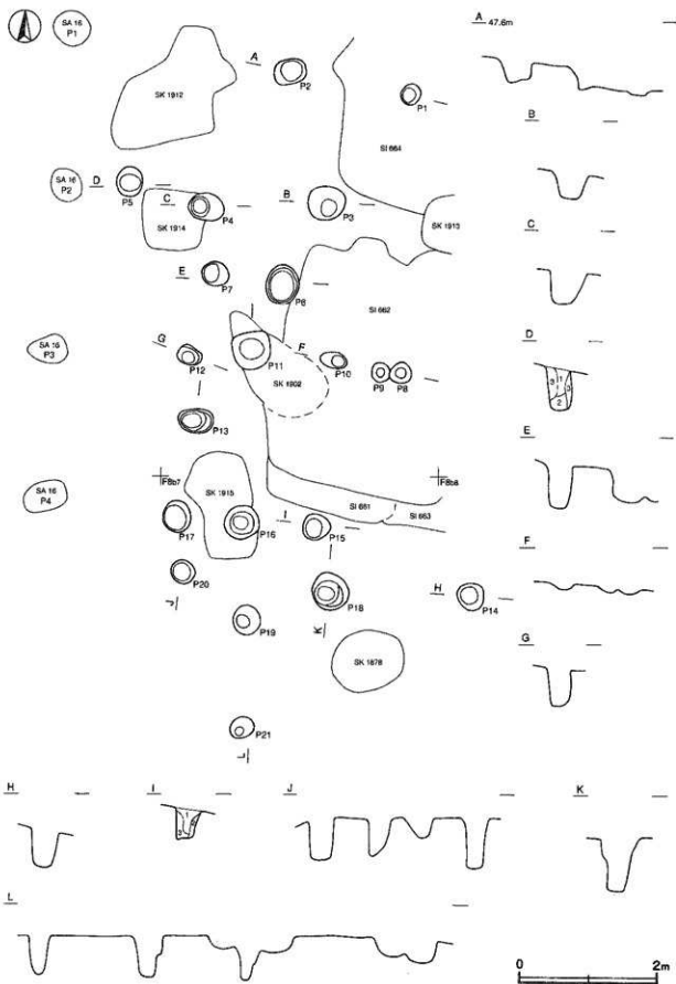
第176図 第43号ピット群実測図
