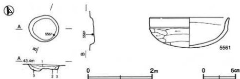
第145図 第1656号土坑・出土遺物実測図
