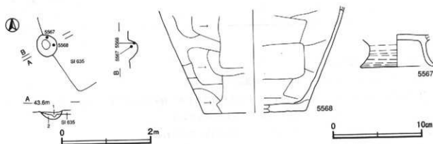
第1745号土坑・出土遺物実測図
