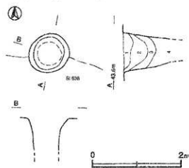
第164図 第65号井戸跡実測図
