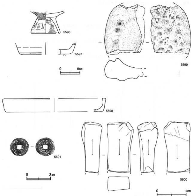
第159図 第2045号土坑出土遺物実測図
