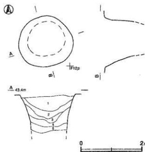
第161図 第62号井戸跡実測図
