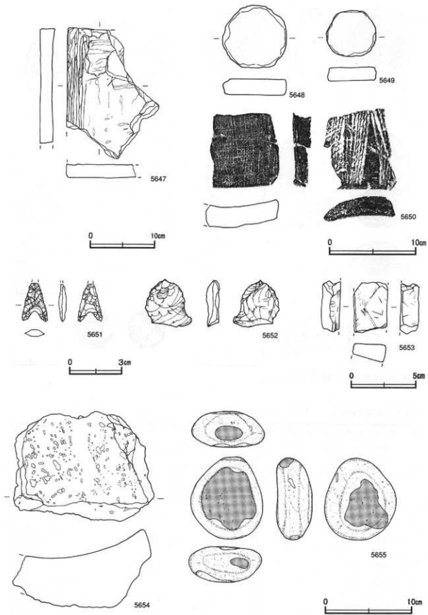
第180图 遺構外出土遺物実測図(2)
