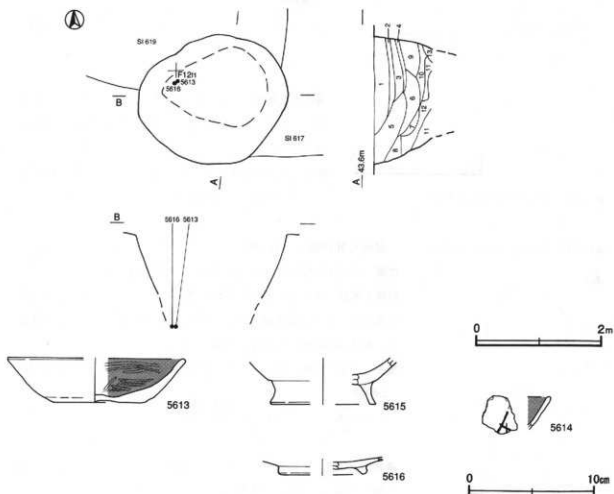
第163図 第64号井戸跡・出土遺物実測図
