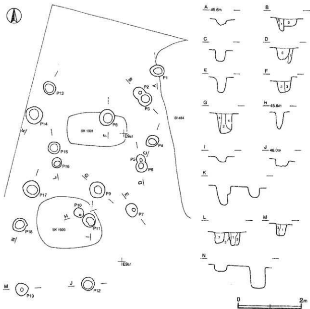
第178図 第45号ピット群実測図
