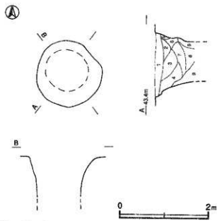
第160回 第61号井戸跡実測図
