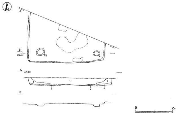
第128図 第668号住居跡実測図
