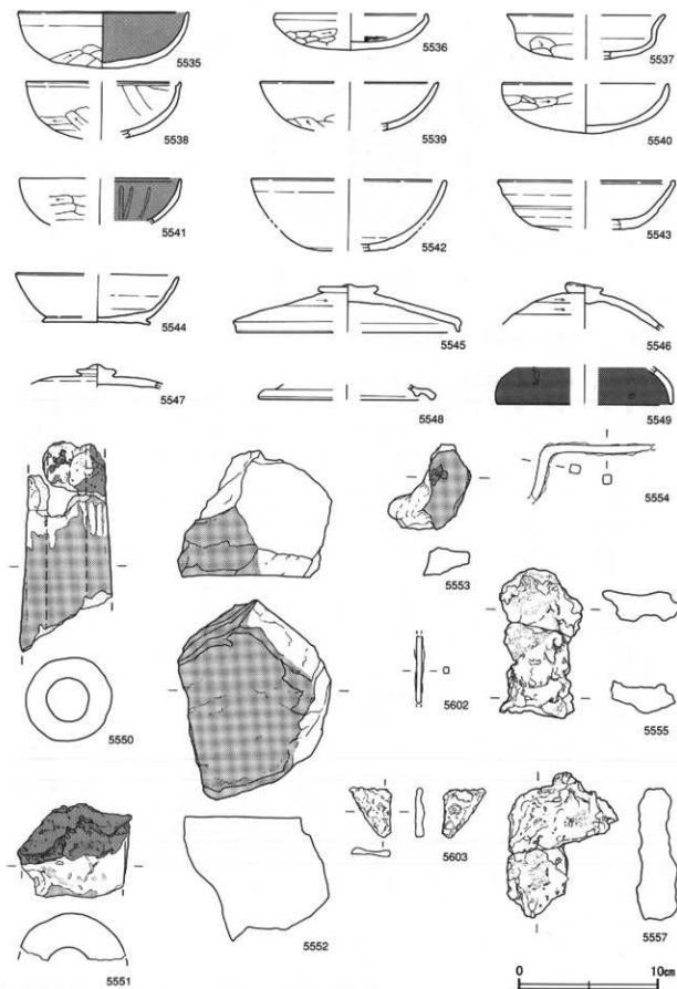
第138图 第2号锻冶工房跡出土遺物実測図(1)
