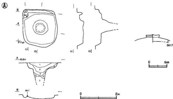
第166図 第67号井戸跡・出土遺物実測図
