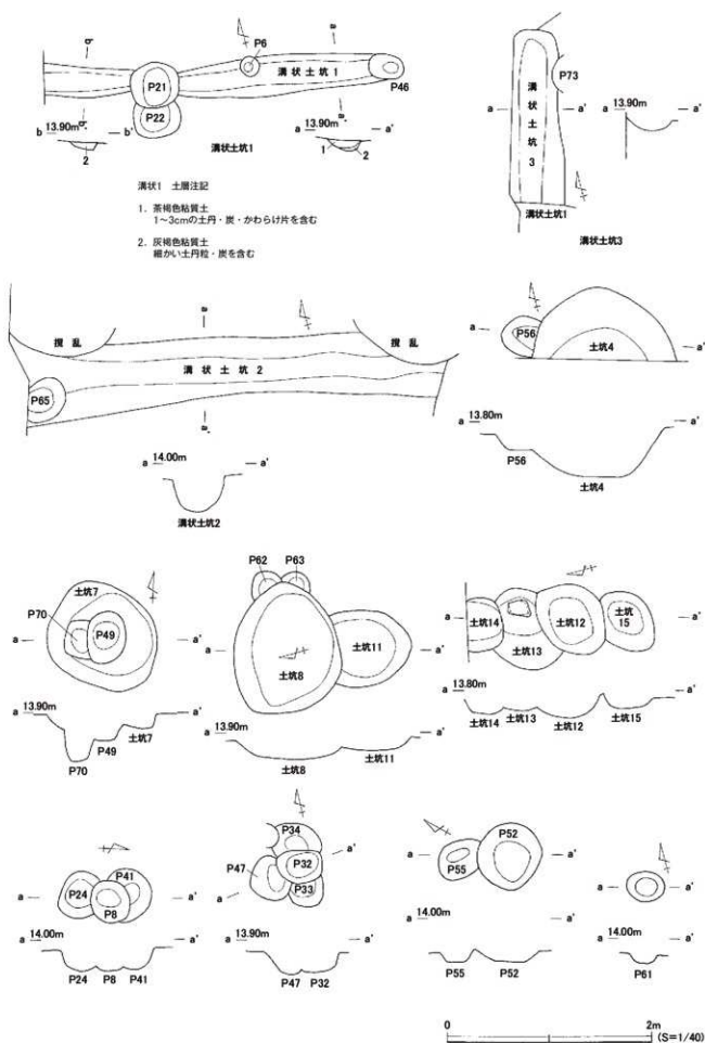
図15 第1面個別遺構図
