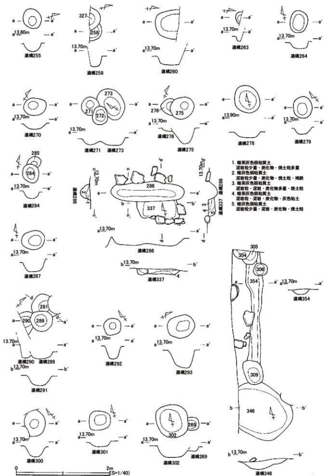
圖20 第3面遺構(1)
