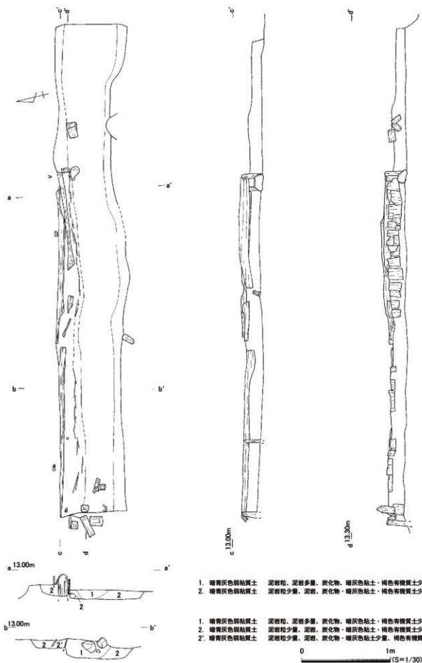
图43 第7面. 遺構480
