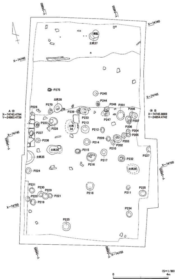
图33 第4面全测图
