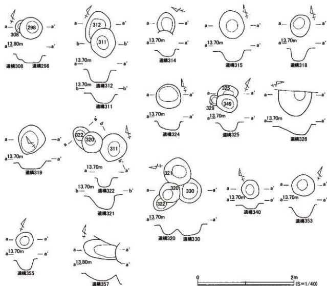
図21 第3面遺構(2)
