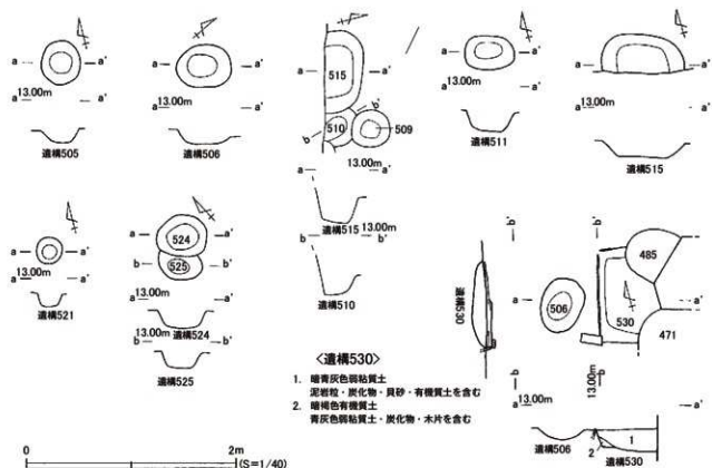
図42 第7面遺構(2)
