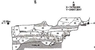
〈トレンチ 西壁セクション図〉
