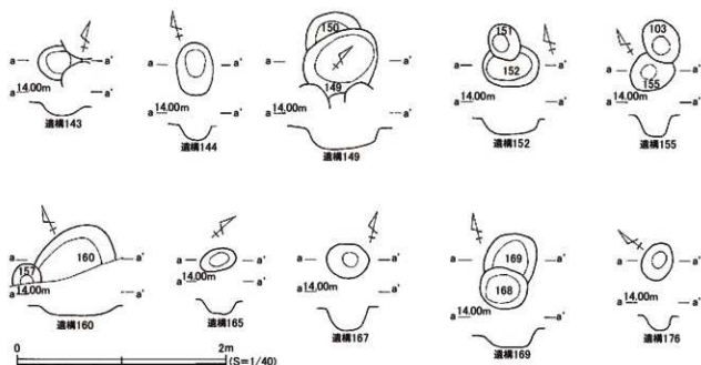
図7 第1面遺構(2)
