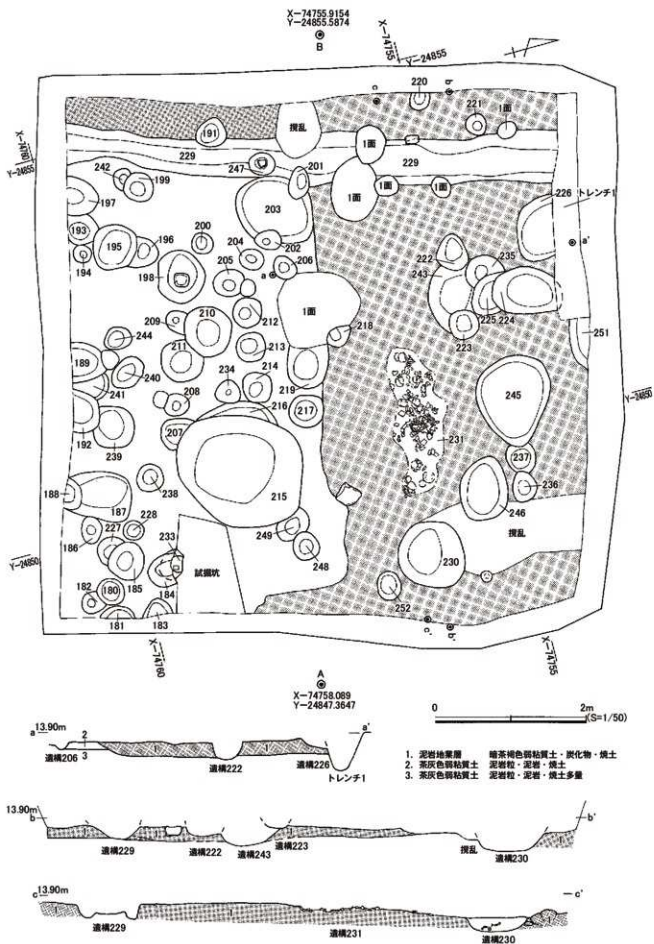
図10 第2面全測図・エレベーション図
