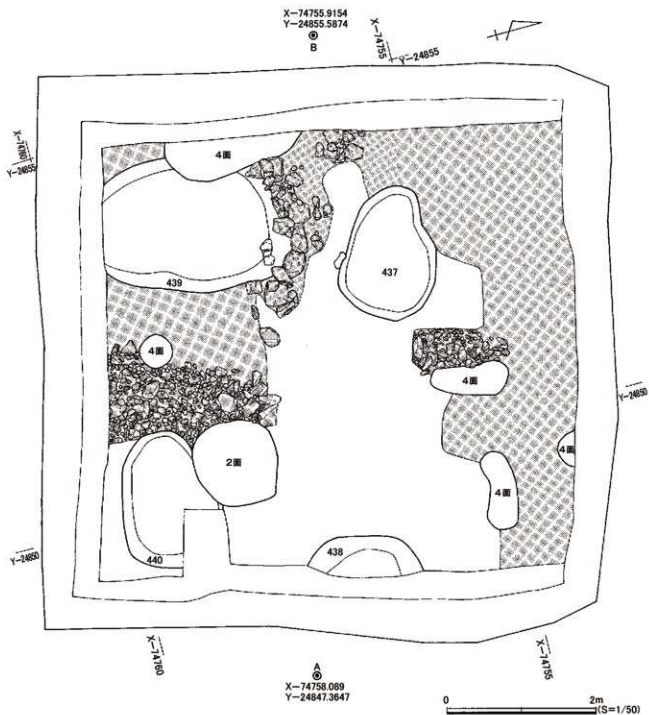
図30 第5面全測図
