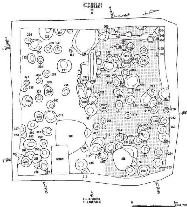
図19 第3面全測図
