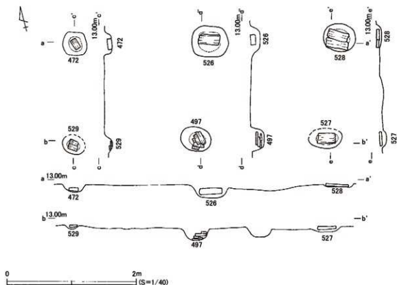
図45 第7面柱穴列
