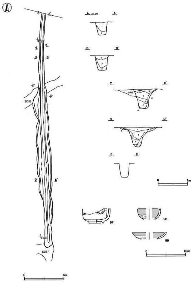
第45图 第56号沟·出土遗物实测图
