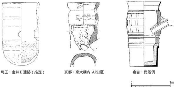
第803図 溶解炉集成図
