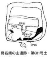
第802図 梵鐘鑄造土坑②(「日本中世における銅鉄の金属生産とその流通に関する研究」より)
