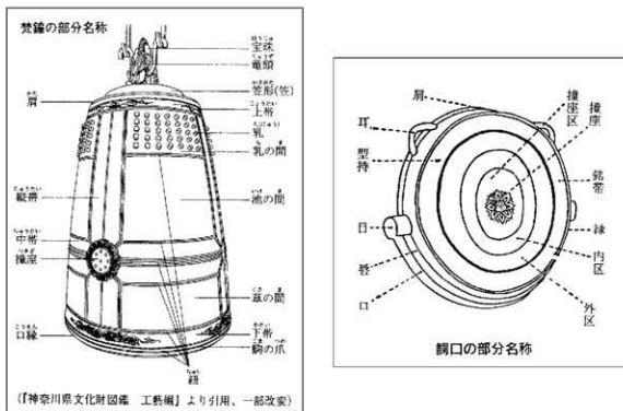
第805図 梵鐘・鯛口の部分名称図（「折りの造形 - 中世霞ヶ浦の金工品 -」霞ヶ浦郷土資料館より）
