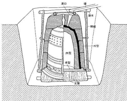
第800図 梵鐘の鑄造状況（「日本中世における鋼鉄の金属生産とその流通に関する研究」より）
