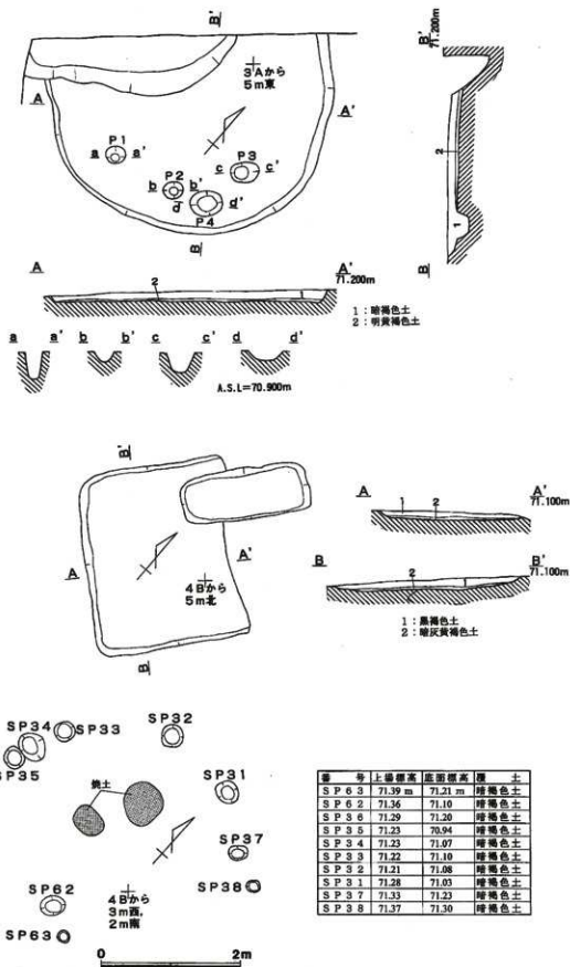
第4図 SB03・SB04・SB05実測図
