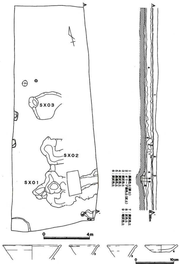
第10图 发掘实测图及び出土遗物实测图
