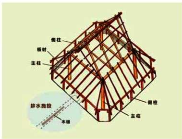
図3 竪穴住居の推定図(川上 貴案)
