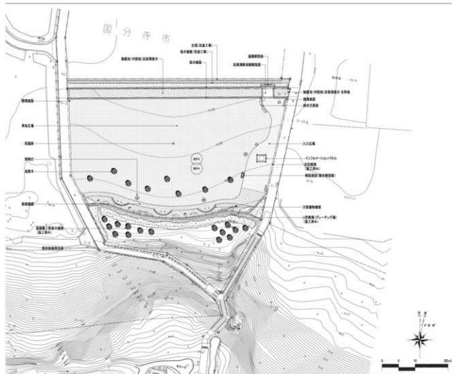
第12図 市立歴史公園 史跡武蔵国分寺跡（僧寺北東地域）整備平面図
