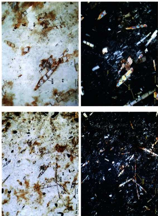
薄片(試料No. 8)の偏光顕微鏡写真(上段は平行ニッケル, 下段は直交ニッケル) 倍率: 左40倍, 右100倍
