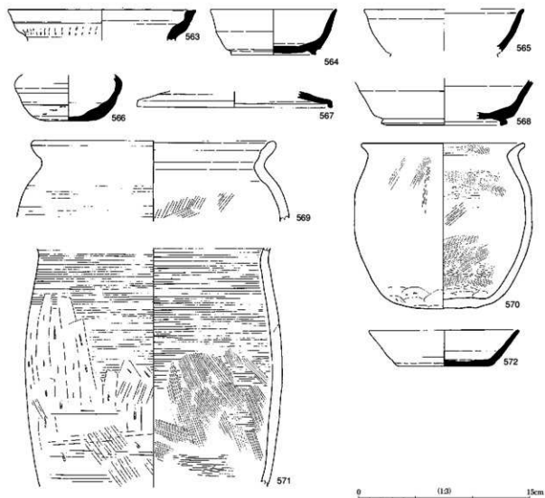
第170図 87ピット等出土遺物実測図
