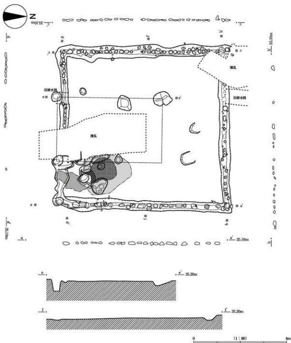
第153図 87SI09実測図
