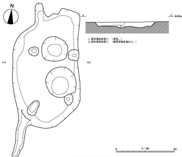
第129図 87SK11実測図
