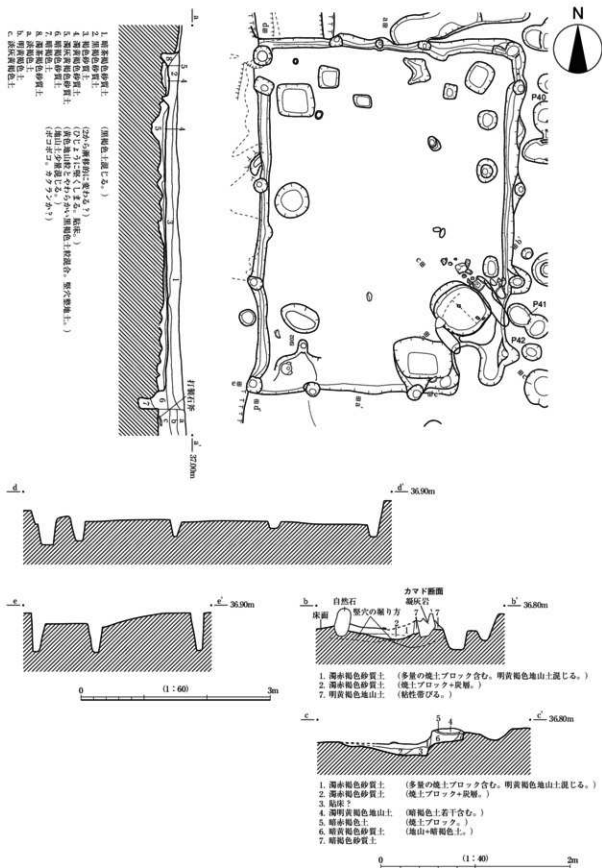
第123図 87S102実測図
