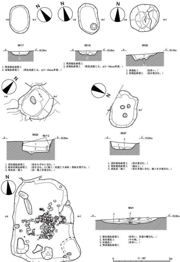
第148図 87SK17・18・21・22・30・37実測図
