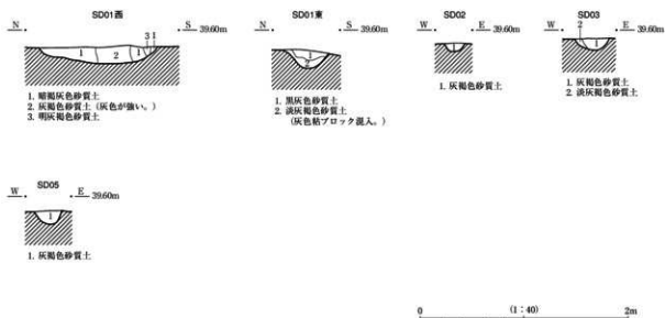
第13図 85SD01・02・03・05実測図
