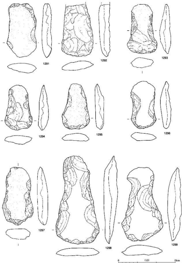
第223図 石製品実測図4
