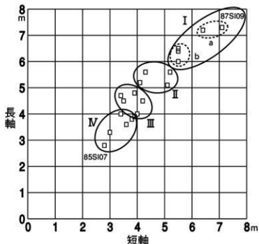
第231図 竪穴建物の規模
