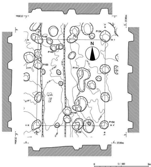
第62図 66SB05実測図
