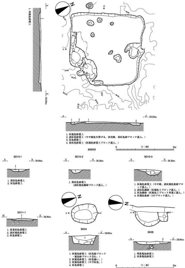
第22図 85SI03・85SK04・05、85SD10・11実測図
