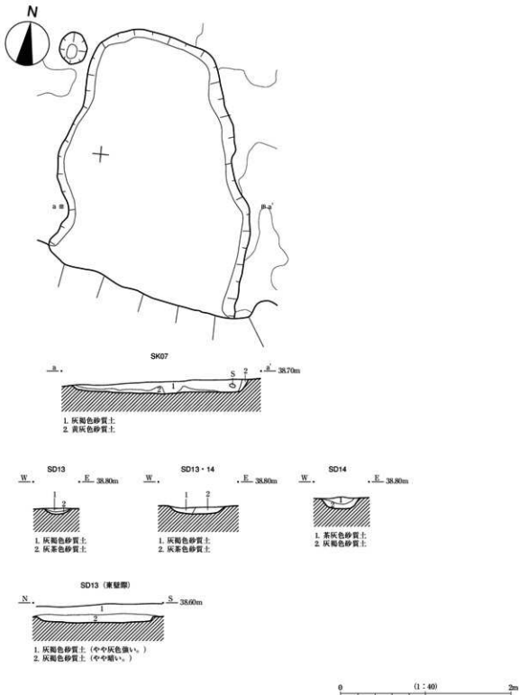
第28図 85SK07、85SD13・14実測図
