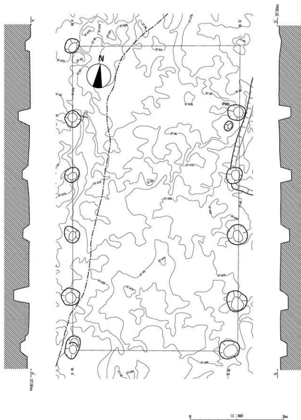
第84図 06SB15実測図
