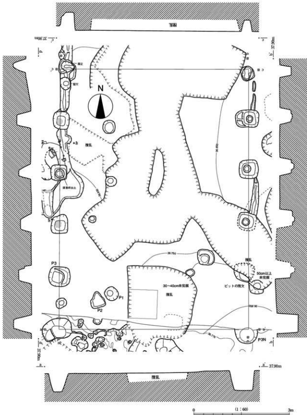
第124図 87SB01実測図
