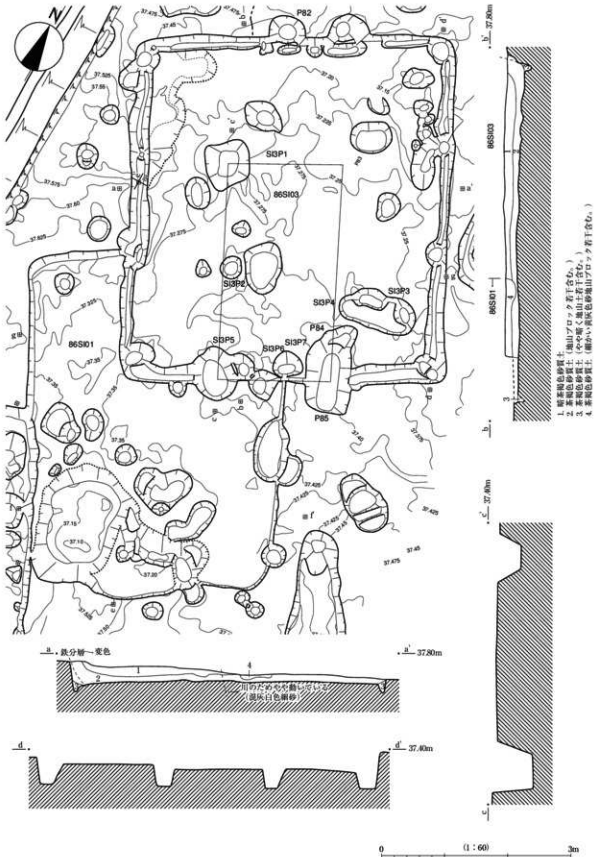
第67図 86SI01・03実測図1
