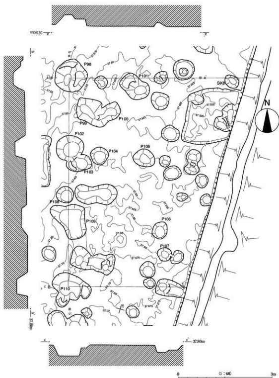
第74図 86SB18実測図
