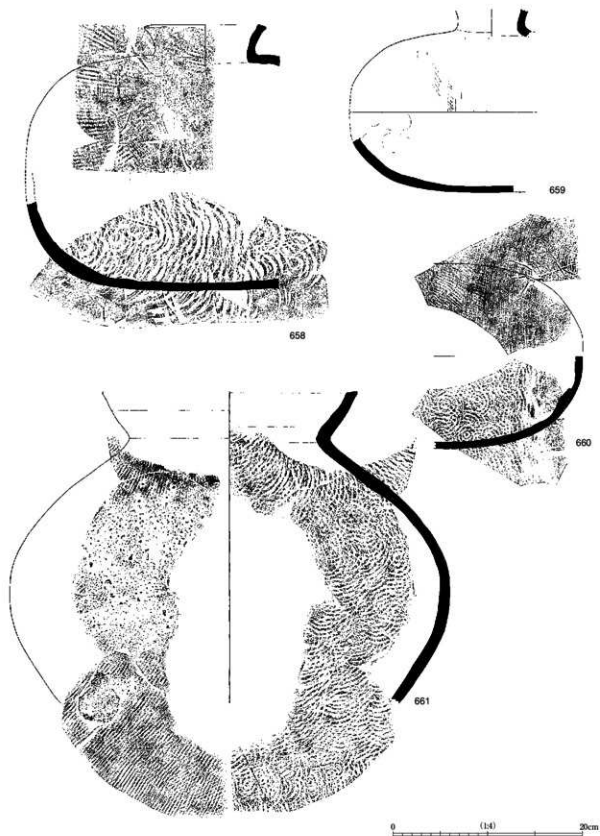
第176図 87大溝 (33ライン) 出土遺物実測図 2
