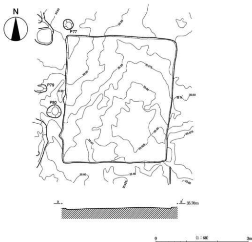
第142図 87SI06実測図
