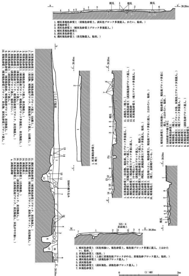
第19図 85SH05・06実測図 2
