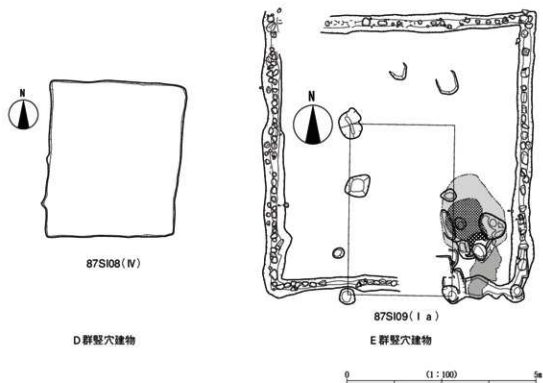
第234図 群別竪穴建物平面図3
