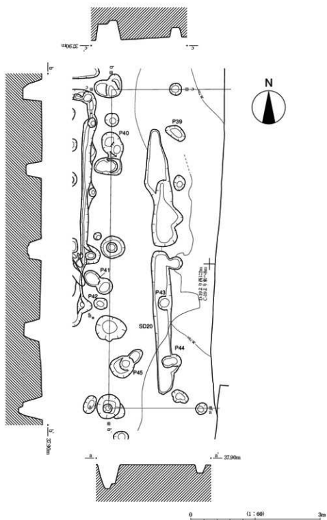
第125図 87SB02実測図
