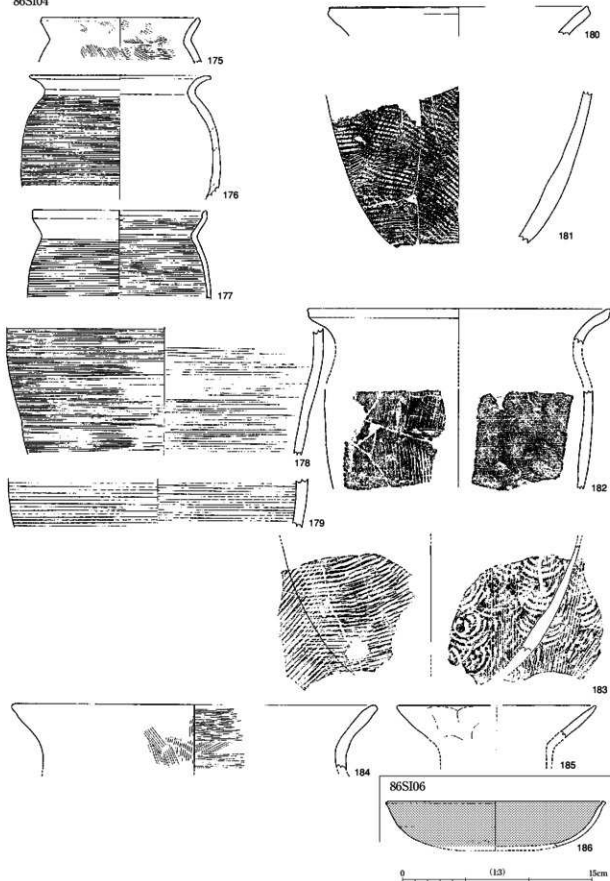
第95図 86SI04・06出土遺物実測図
