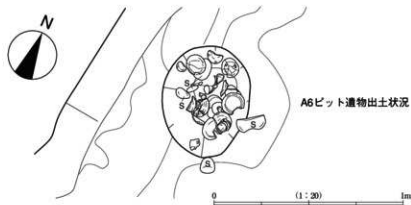
第25図 85SB01、A6ピット実測図
