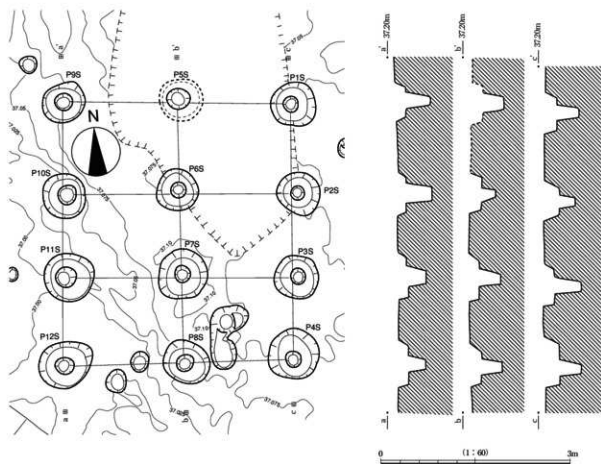
第69図 86SB21実測図
