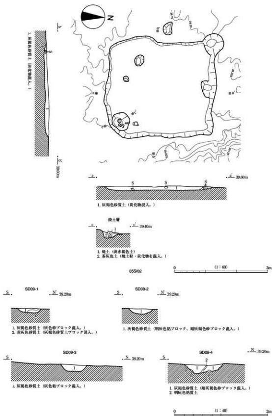
第20図 85SI02、85SD09実測図
