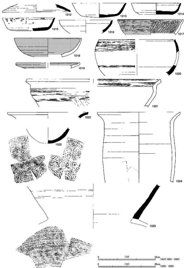
第206図 87包含層出土遺物実測図1
