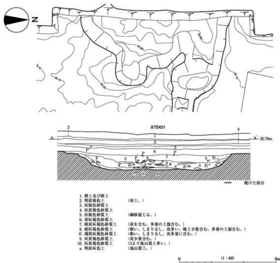
第146図 87SX01実測図
