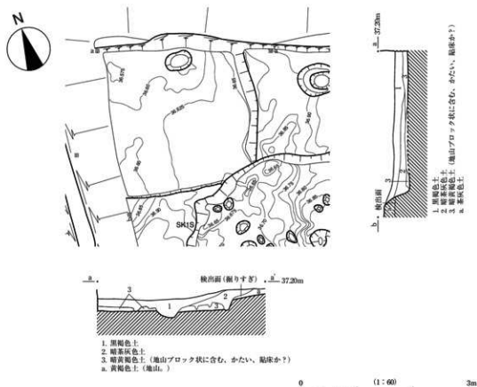
第68図 86SH12実測図
