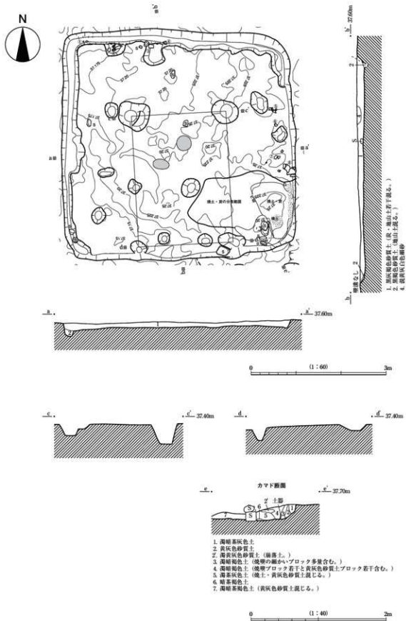
第69図 B6SI04実測図
