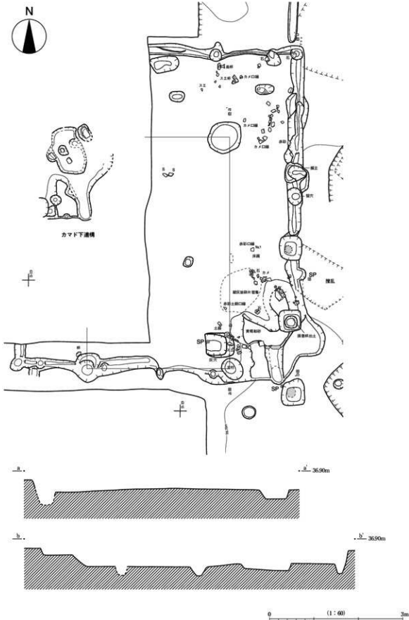
第127図 87SI01実測図1
