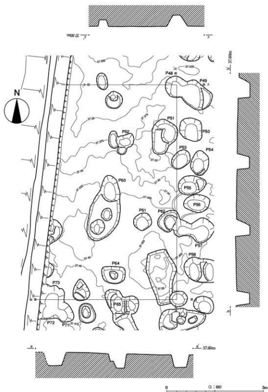
第80図 86SB20実測図
