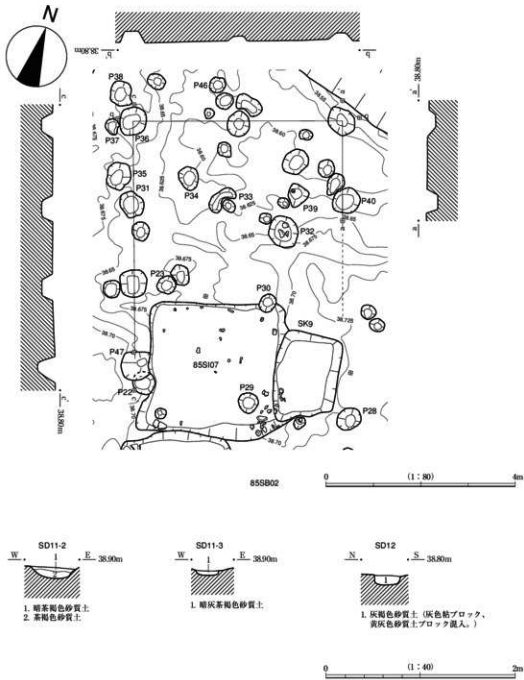
第26図 85SB02、85SD11・12実測図
