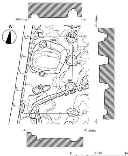
第72図 66SB09実測図
