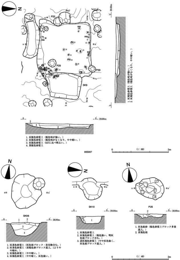
第24図 85S107、85SK06・10、85P25実測図
