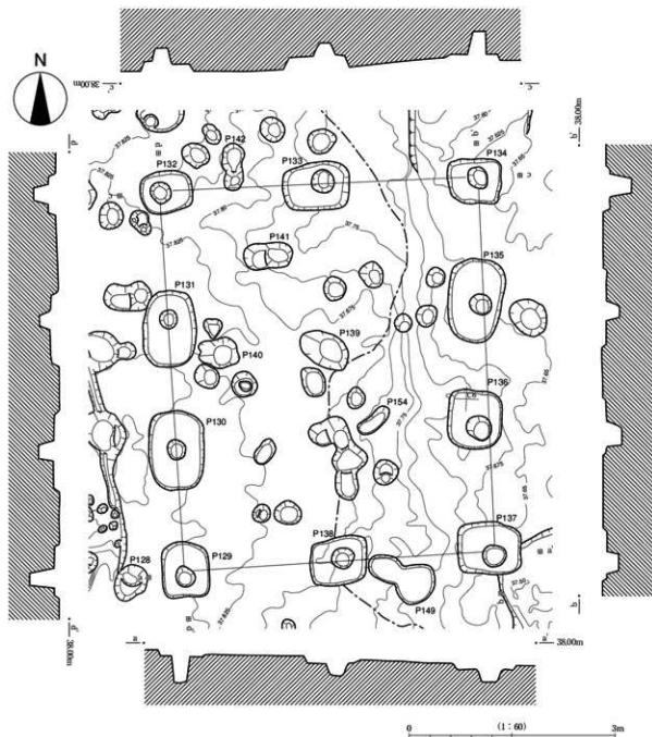
第56図 86SB02実測図
