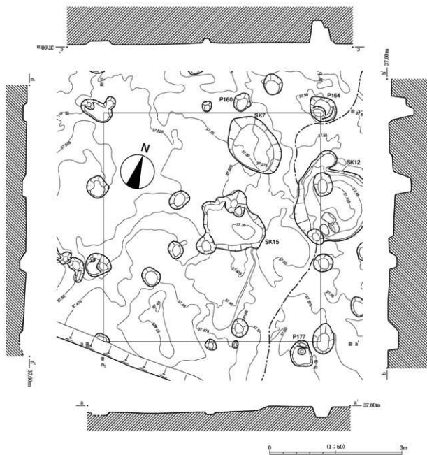
第61図 86SB03実測図
