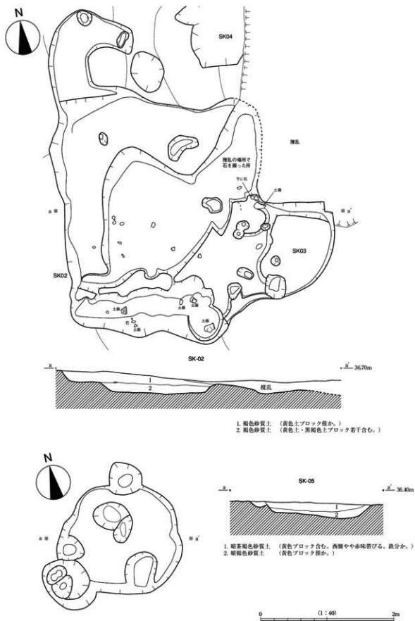
第132図 87SK02・05実測図
