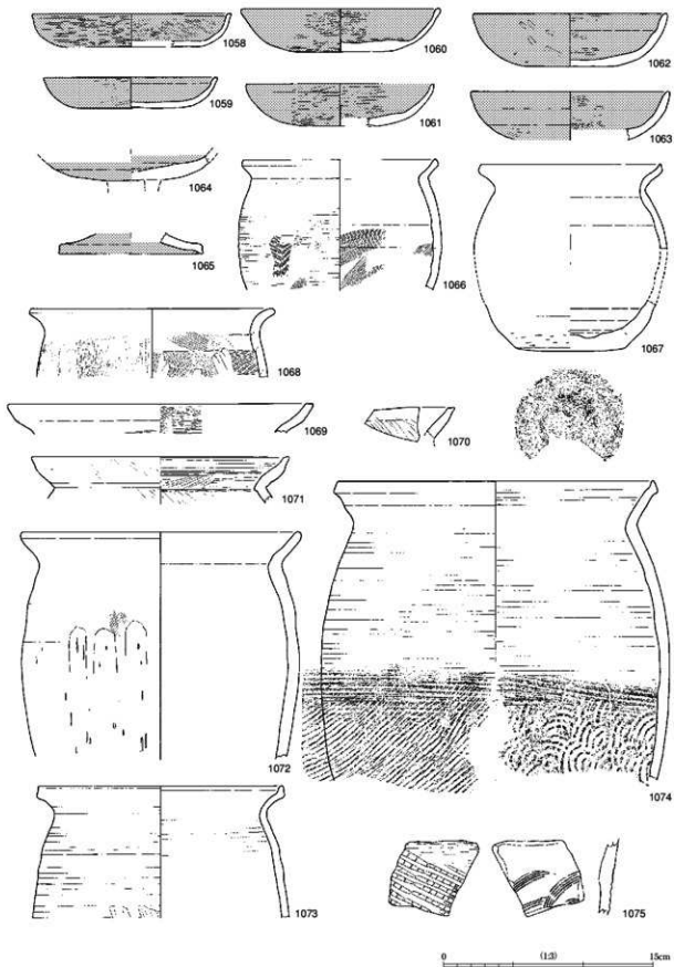
第208図 87包含層出土遺物実測図3
