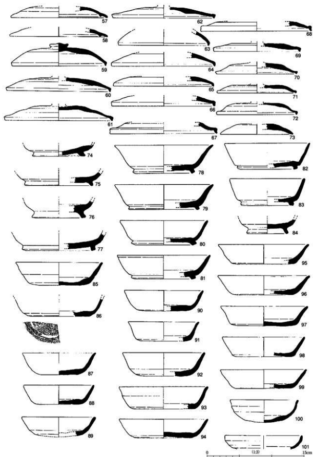
第37図 85包含層出土遺物実測図1
