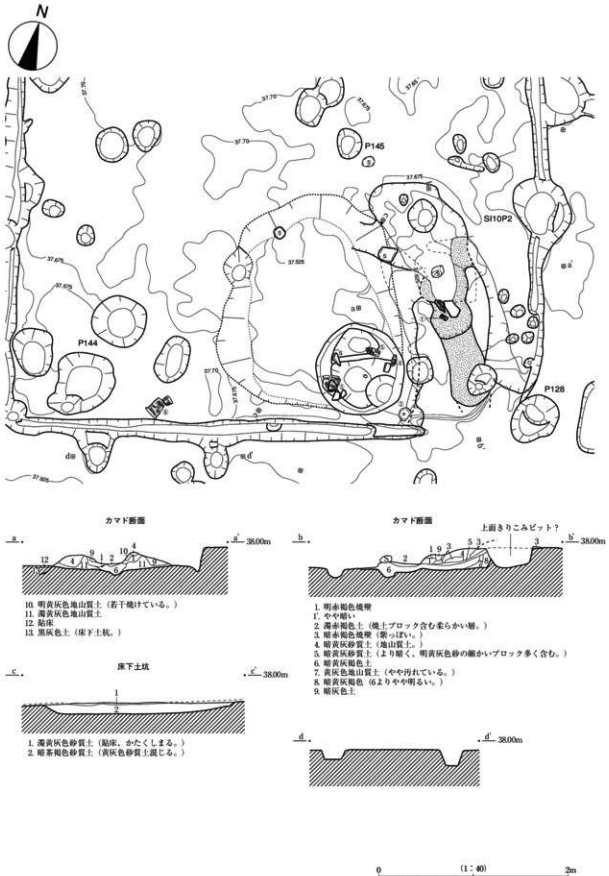
第53図 86SI10実測図 2
