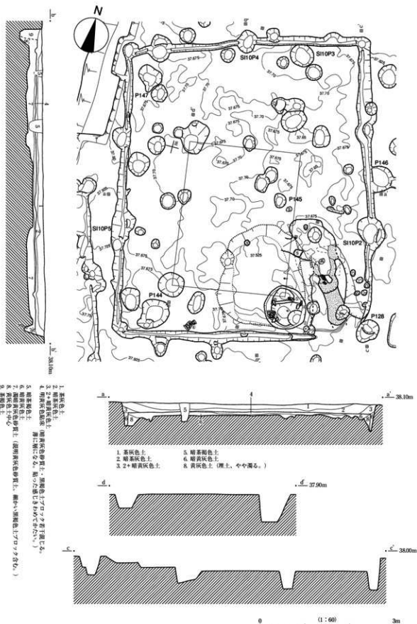
第52図 86SI10実測図1
