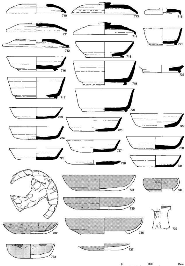
第180図 87大溝 (36ライン) 出土遺物実測図1
