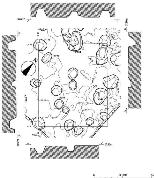
第63図 86SB06実測図
