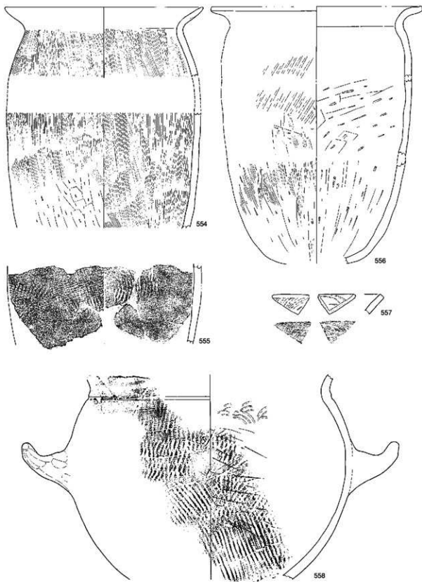
第168図 87SX01出土遺物実測図3
