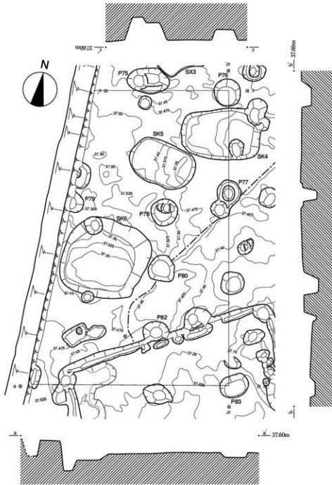
第73図 86SB10実測図
