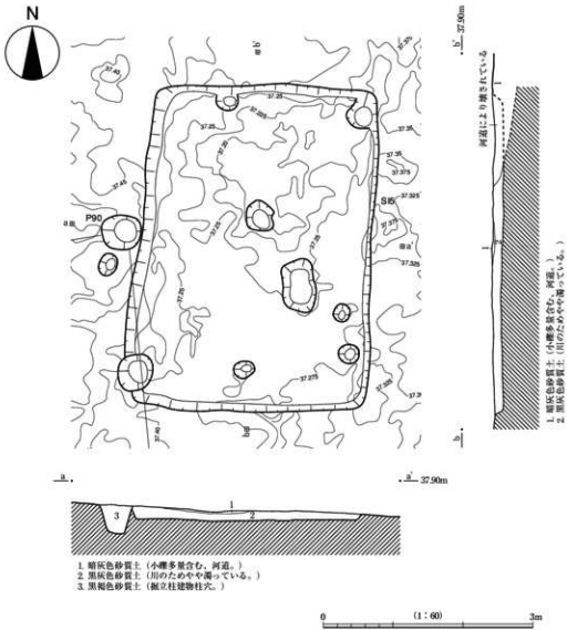
第82図 86SI05実測図
