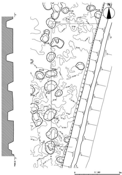
第65図 86SB17実測図
