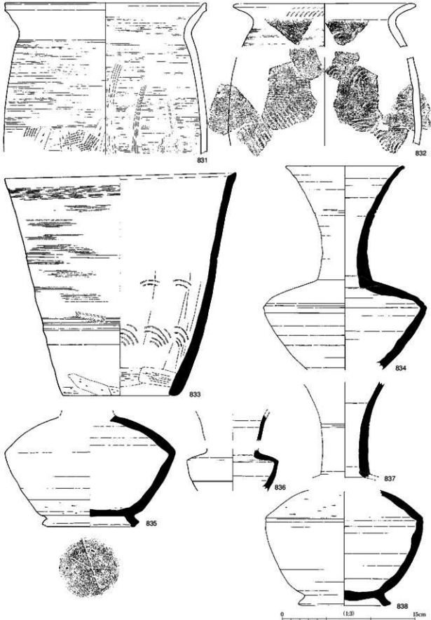
第191図 87大溝(38ライン)出土遺物実測図2
