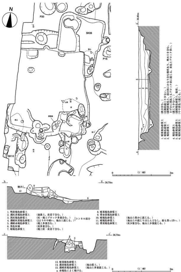
新134図 87S103実測図
