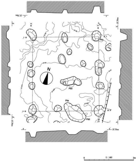
第79図 86SB16実測図
