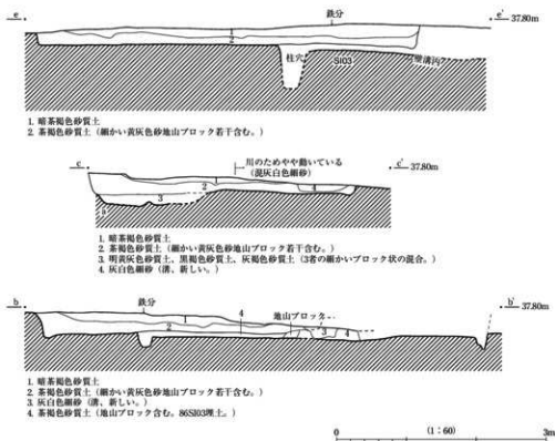
第68図 86SI01・03実測図2
