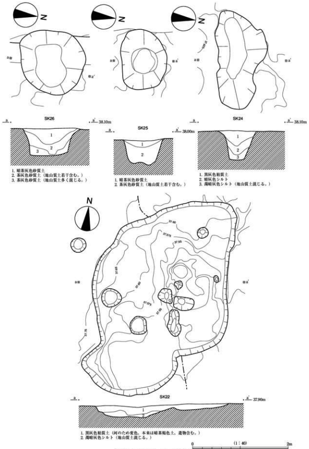
第50図 86SK22・24・26実測図
