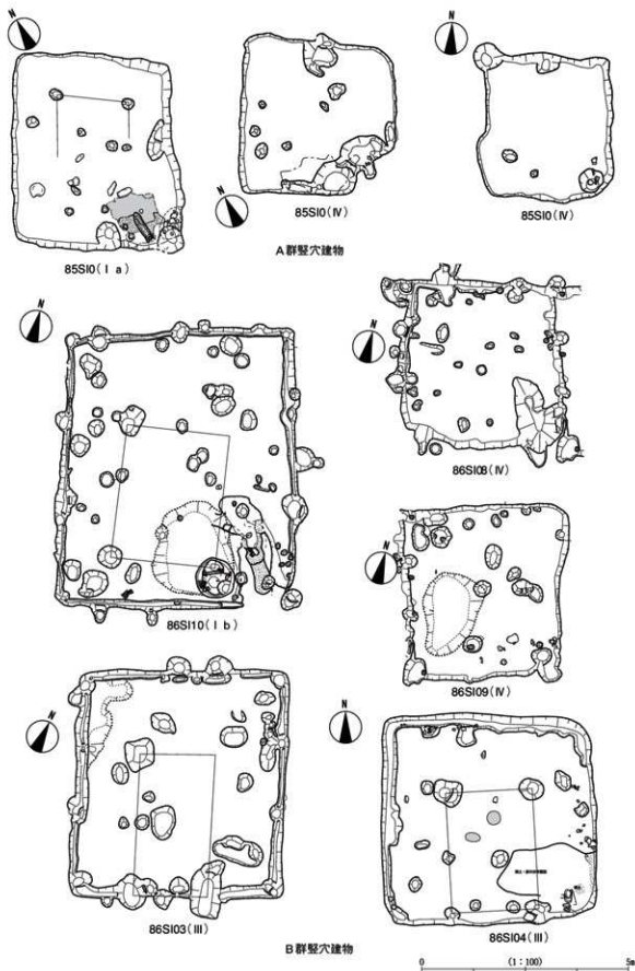
第232図 群別竪穴建物平面図1
