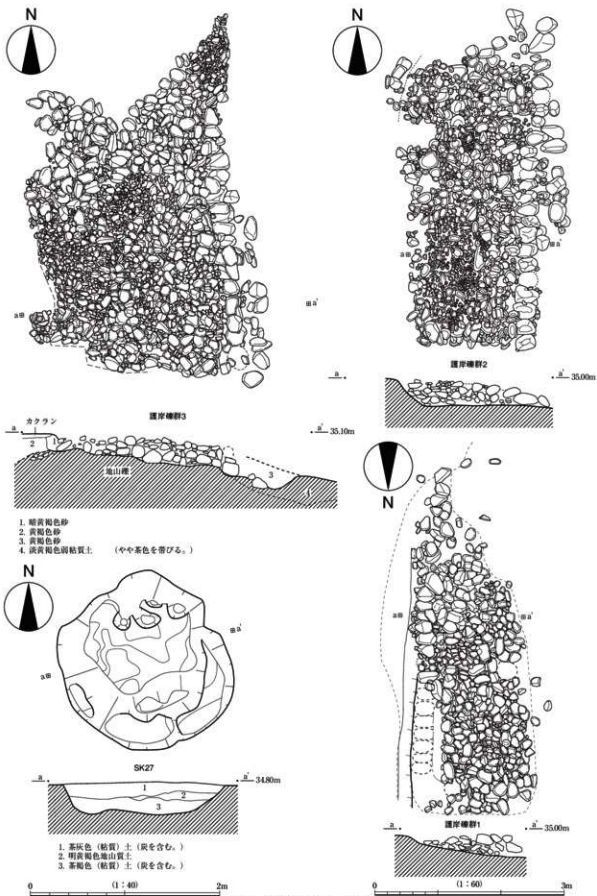
第151図 護岸礫群、87SK27実測図
