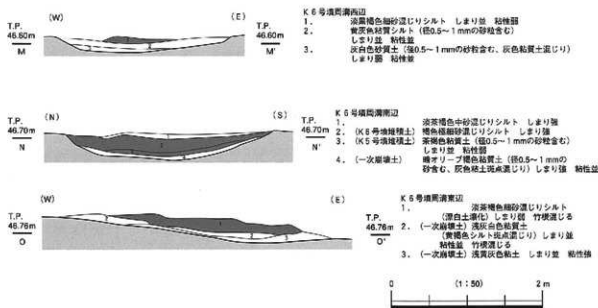
第25図 K6号墳 周溝断面図
