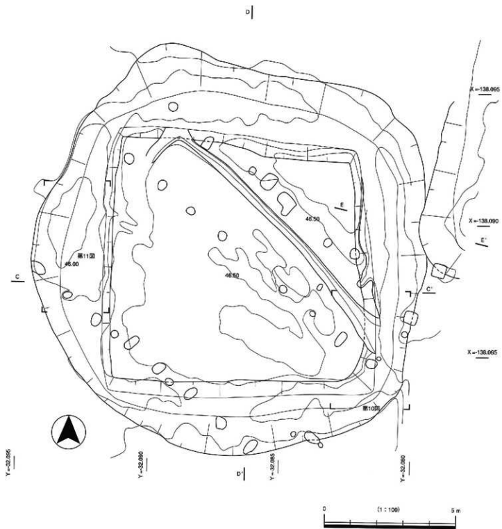
第9图 K2・K4号墳 平面图
