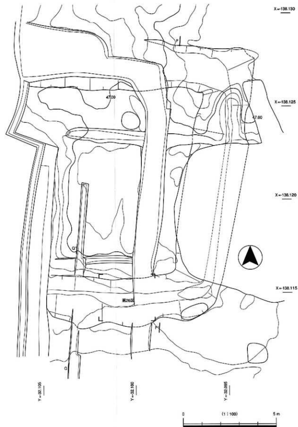
第29図 K 7号墳 平面図
