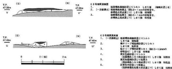
第36図 K 8号墳 周溝断面図
