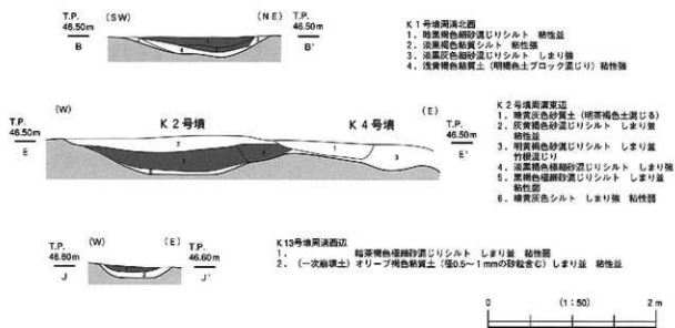
第6図 K1・K2・K13号墳 周溝断面図
