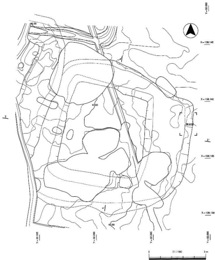
第31図 K10・K12号墳 平面図
