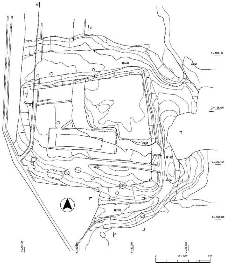
第15図 K3号墳 平面図
