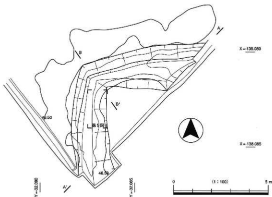
第4図 K1号墳 平面図
