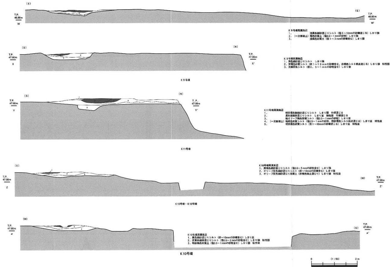
第34図 K 9～K 12号堤 断面図
