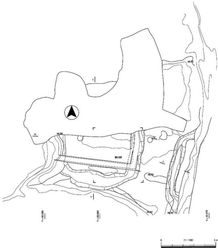
第21图 K5・13号墳 平面图
