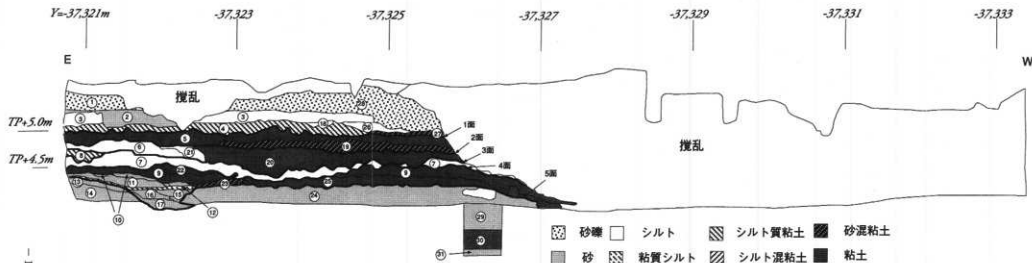
図 18 Pit.1 南壁断面図
