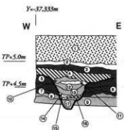
図31 溝115北壁断面図
