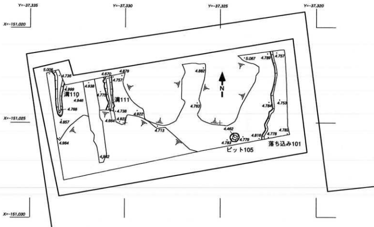
図22 Pit.1 第1面、遺構平面図
