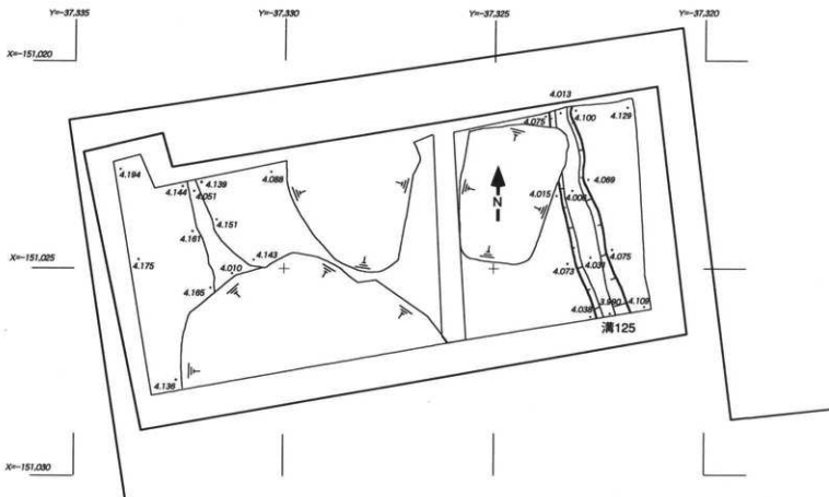
図51 Pit.1 第5面、遺構平面図
