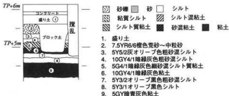
図84 土取り穴北壁 柱状断面図
