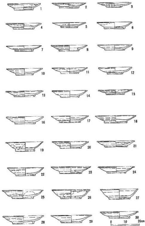
图版6 皿 (1:4)
