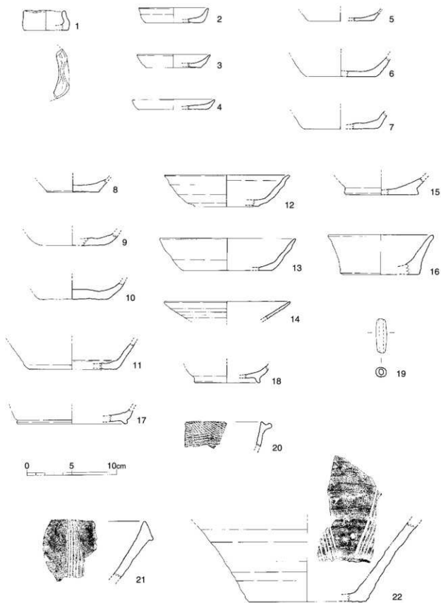
第5图 11·12层出土遗物实测图(1/3)
