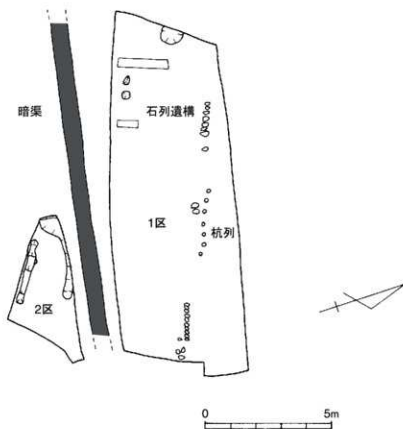
第2図 調査区遺構配置図 (1/150)
