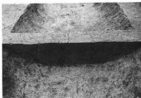
RG115埋土断面(南から)
