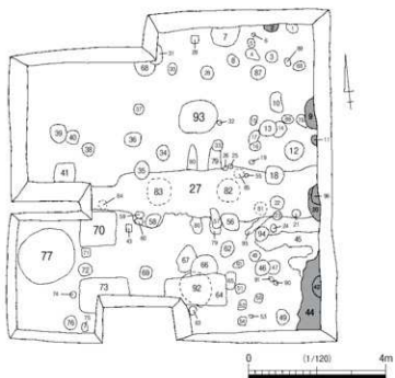
図4 遺構配置図
