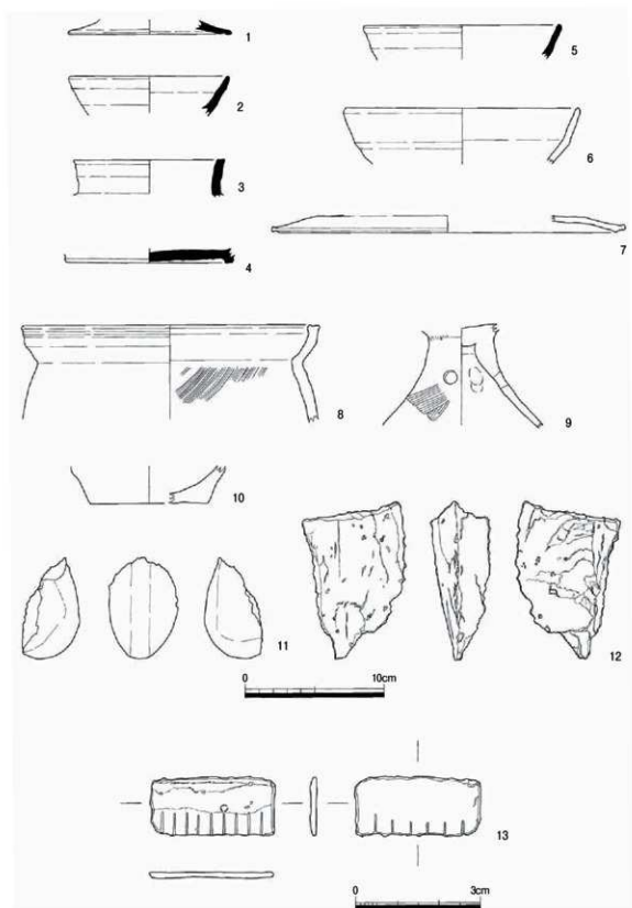
图4 遗物实测图
