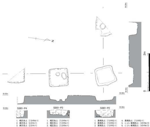
図3 SB01全体図・土層断面図
