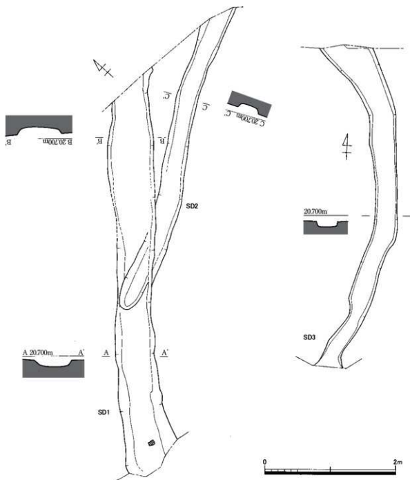
第33図 1～3号溝状遺構実測図 (S=1/40)
