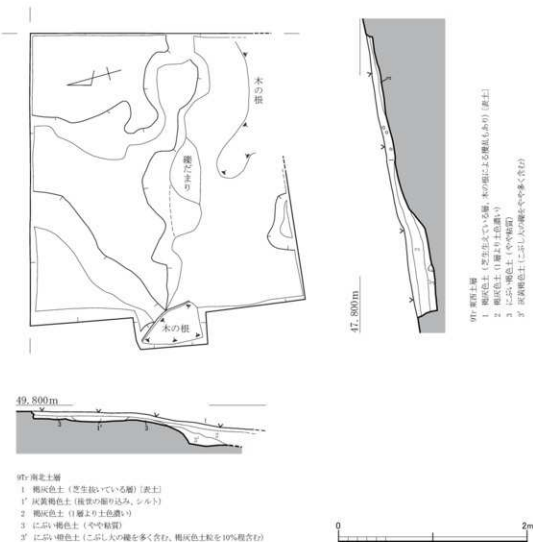
第13図 津古1号墳9トレンチ平面図・断面図 (S=1/40)
