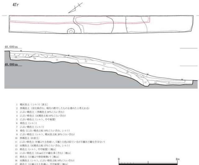
第8図 津吉1号墳4 トレンチ平面図・断面図 (S=1/40)
