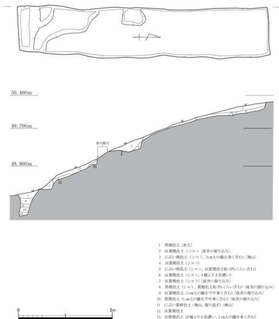
第6図 津古1号墳2トレンチ平面図・断面図 (S=1/40)
