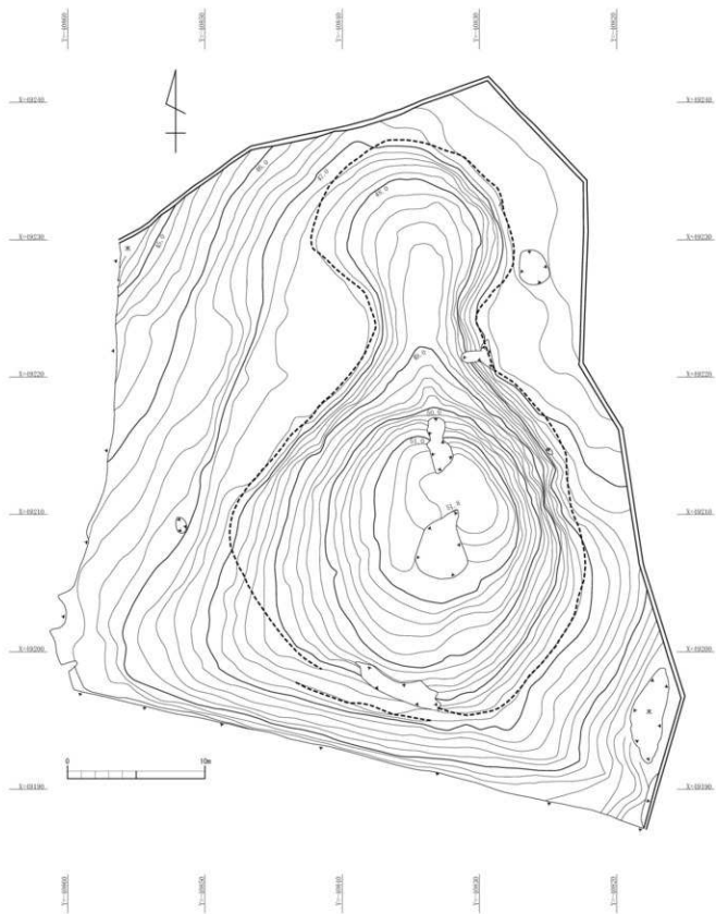
第3図 津古1号填測量図 (S=1/300)
