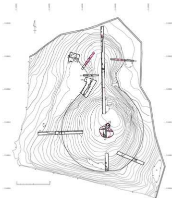
第15図 津古1号墳墳丘復元図(S=1/500)
