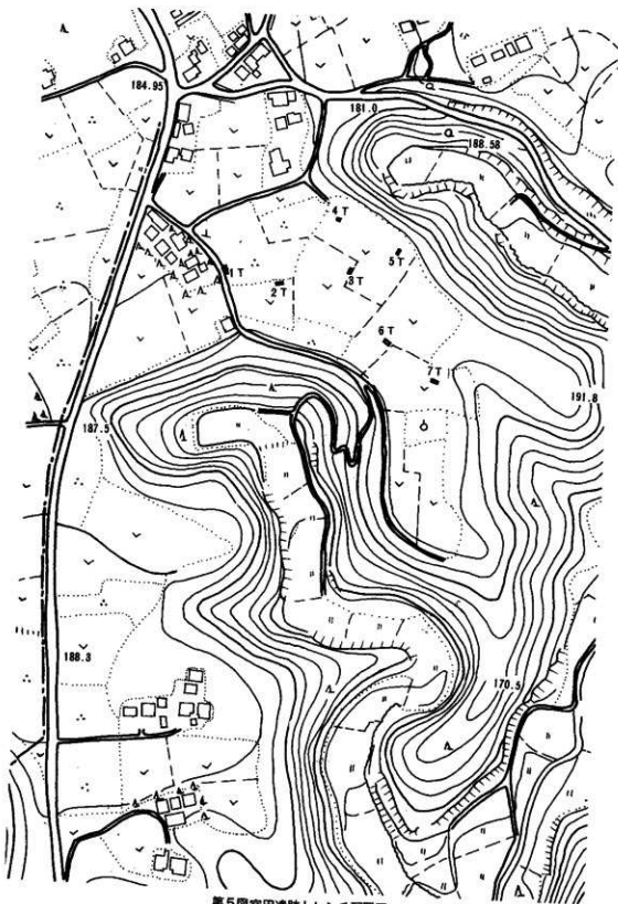
第5回宮田遺跡トレンチ配置図
