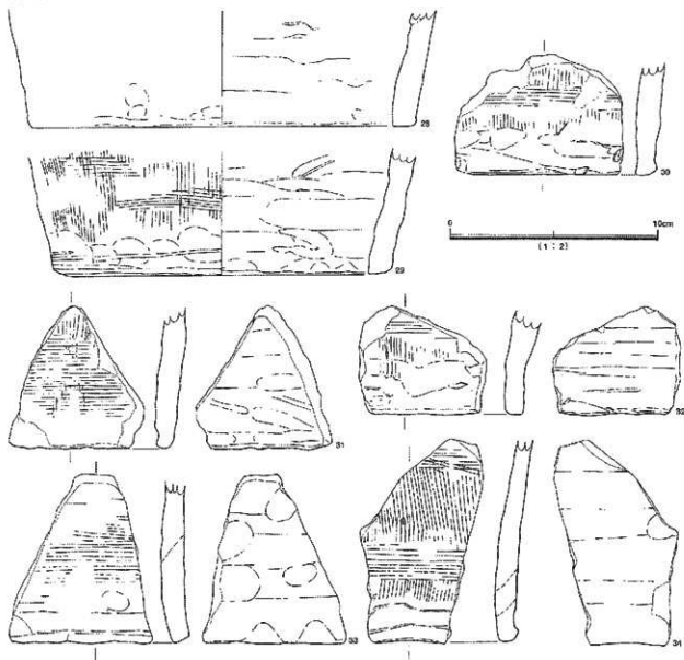
第30図 円筒埴輪実測図(1)
