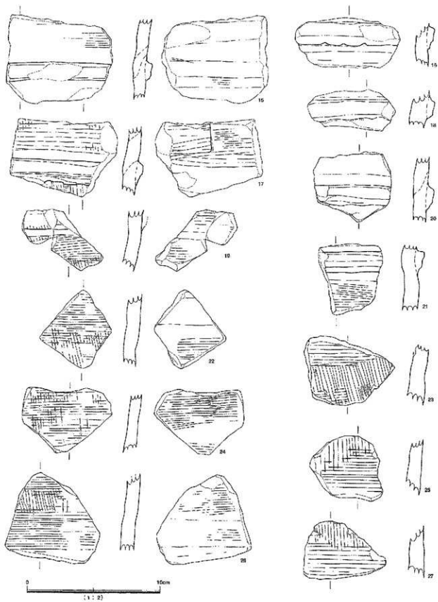
第32圖 円筒槍尖測圖(3)
