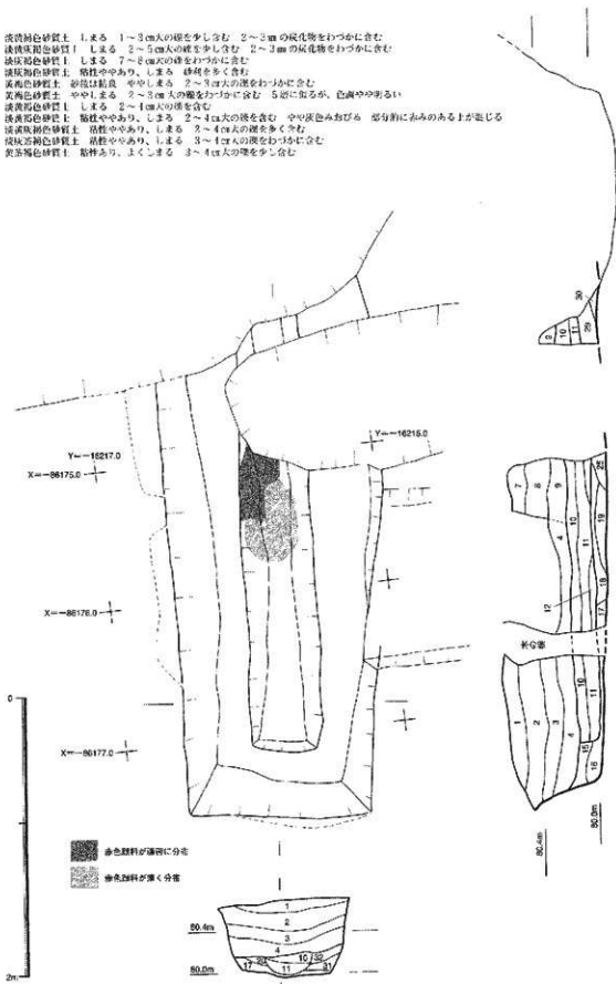
第28図 埋葬施設 平面図・断面図
