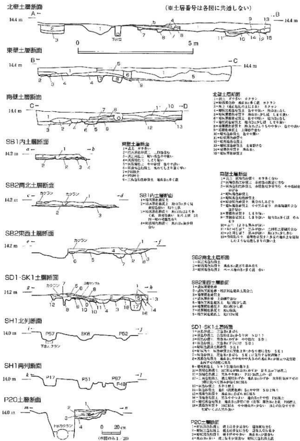
図4 土層断面図
