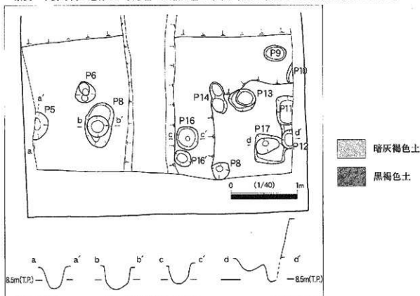
第9図 調査区南半平面図及びピット断面図
