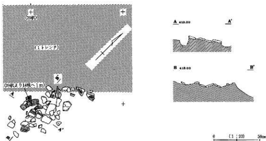
図6 遺物集中部1 (上面) 平面図・断面図
