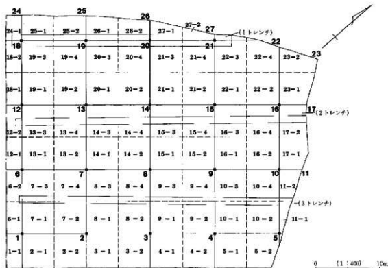
図3 グリッド配置図
