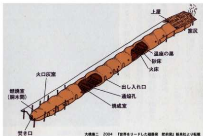
第3図 連房式登窯模式図
