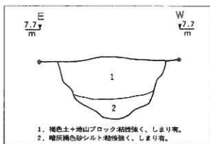
第7図 SK01断面図 (S=1/15)
