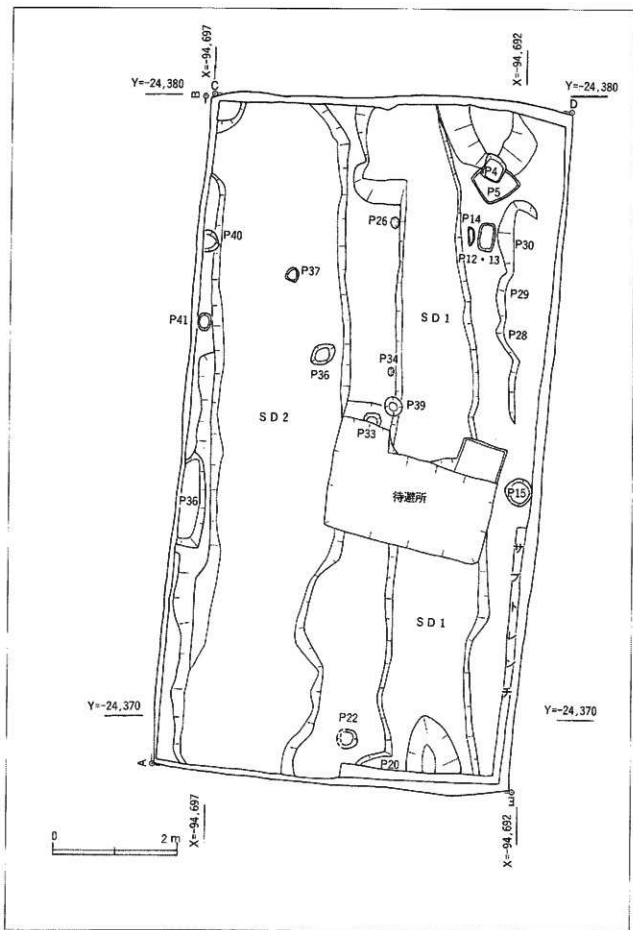
第11図 遺構平面図 (S=1/60)
