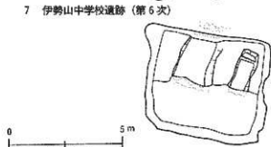
第17図 待避所の構造と調査事例
