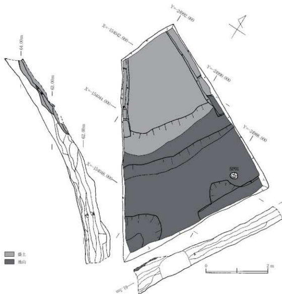
図4 第13調査区平面図・断面図 1:60
