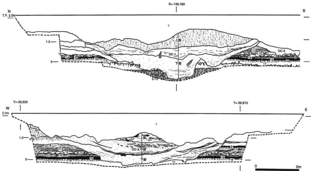
図5 調査地東壁断面(上)および北壁断面(下)
