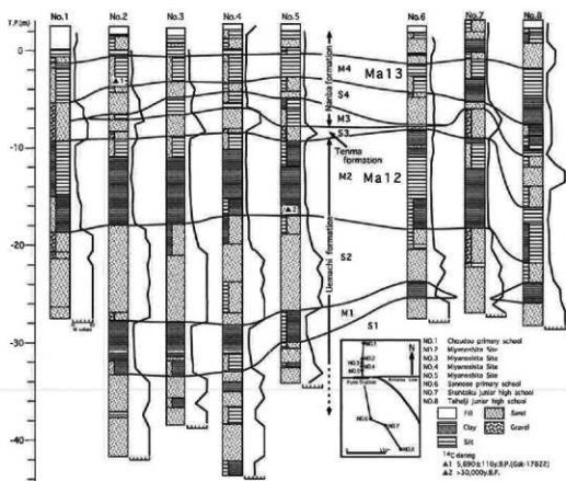
図2 近鉄布施駅周辺のボーリング柱状図の層序対比
