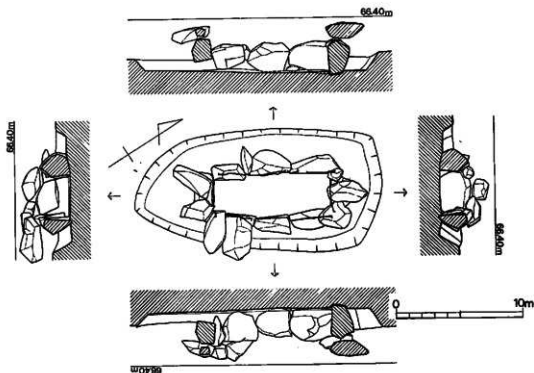
第66図 都地W-4号墳石室実測図 (1/30)
