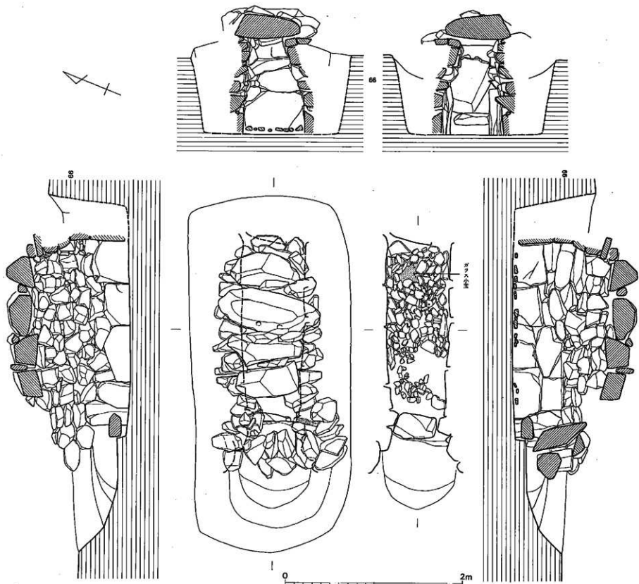
第57图 郝地W-1号横石室实例图(1/30)
