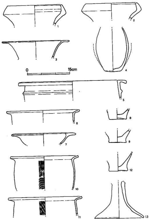
第36图 西区出土土器类图(1/4)
