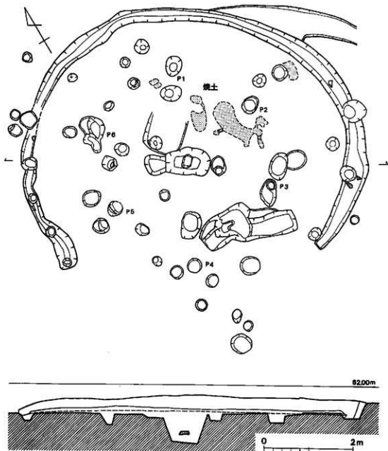
第33図 第25号住居跡実測図 (1/60)
