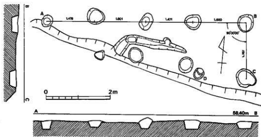
第15图 第7号圆立柱建物实测图(1/60)
