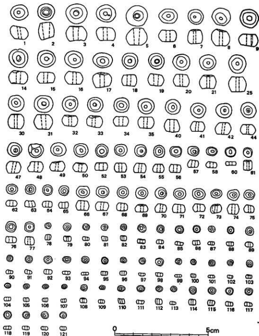
第60图 都地W-1号堆出土小玉实剖图 (1/1)
