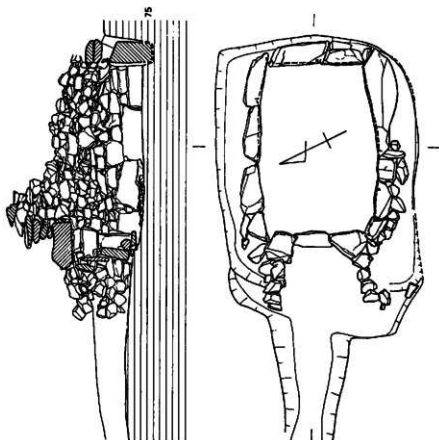
第86図 沙井掛1号墳石室 (1/60)
