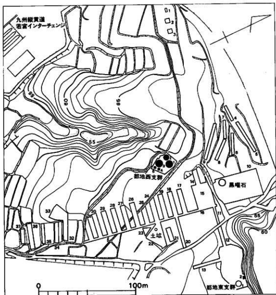
第36図 都地遺跡トレンチ配置図 (1/2,000)
