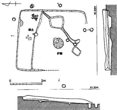
第31図 第24号住居跡実測図 (1/60)
