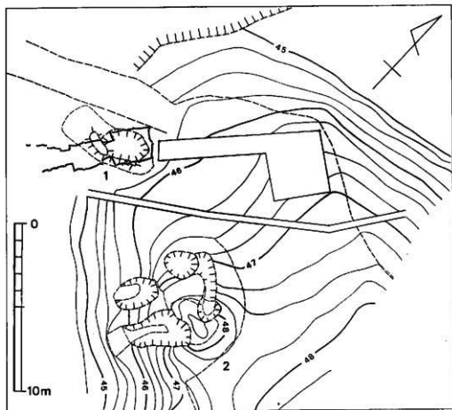
第79図 平原古墳群地形実測図 (1/200)
