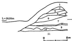
第8図 墳丘断面図 (S=1/80)
