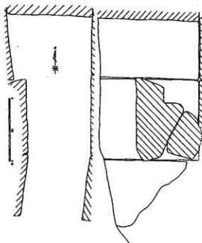
2. 石室断面図 (川上ほか 1972)
