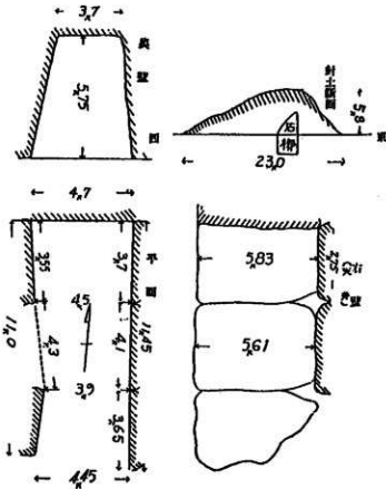
4. 石室実測図 (内務省 1927)
