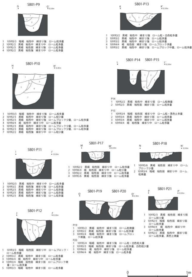
第 70 図 掘立柱建物跡 SB01 柱穴セクション②
