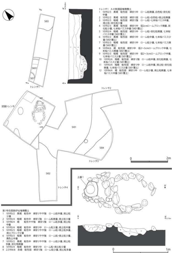
第53図 軍民坂遺跡(第2地点)の遺構配置と第1号住居跡炉址
