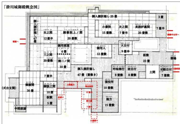
〔竣工平面図〕(復元図面) (「静岡県指定文化財 掛川城御殿修理工事報告書」に加筆)
