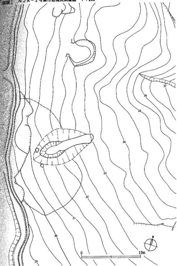
图版 I NJA-2号窟付近現況測量圖 1:200
