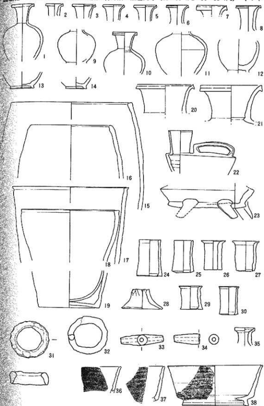
圖版Ⅺ 小型長頸瓶・平瓶・土鐘・特殊品・窯道具等 (33~35 1/2・36~38 1/3) 1:4
