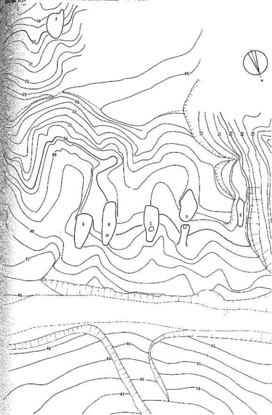
圖版 XIV NK 1-1 群附近現況測量圖 1 : 300
