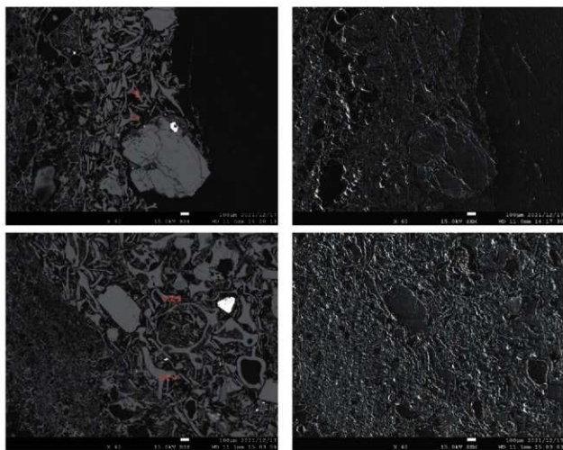
第 46 図 H-1 の BSE 像と SEM 像および測定ポイント
