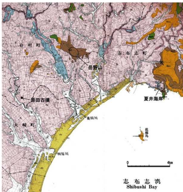
第 50 図 原田古墳・夏井海岸・岳野山の位置と志布志地域の地質（『鹿児島県地質図より作成』）
