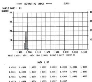
第 47 図 H-1 火山ガラスの屈折率
