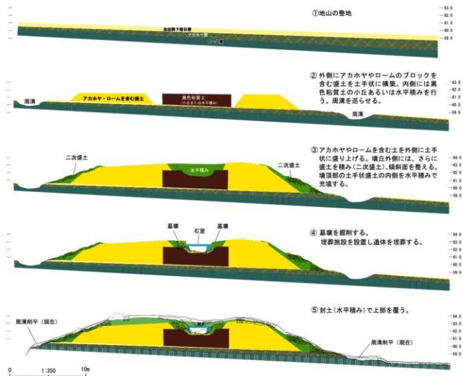
第 52 図 原田古墳墳丘構築手順想定図
