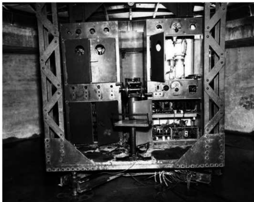
第68図 タチ3号送信機 地下部分（米国立公文書館）1945年10月30日撮影 工藤洋三氏提供 名古屋で撮影されたもの
