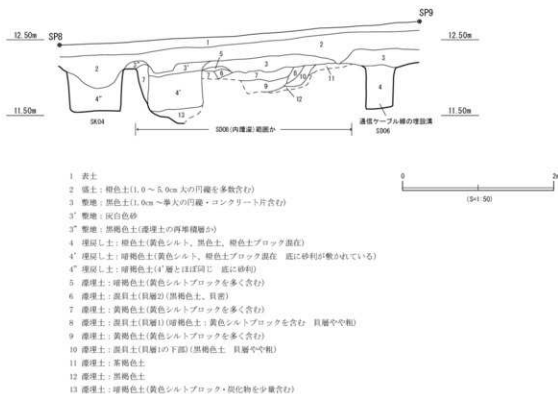
第13図 第49次土層図 (A区 東壁 (SD08))
