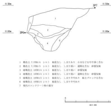
第17図 第49次土層図 (A区SD01)
