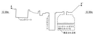
第55図 電波標定機受信所 (試掘調査)
