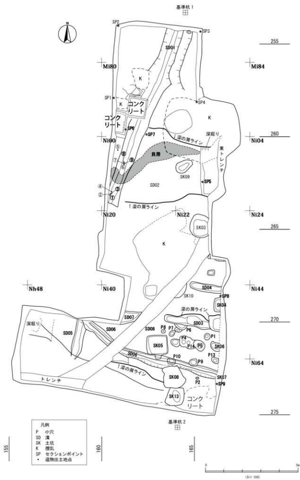
第11図 第49次遺構全体図 (A区)
