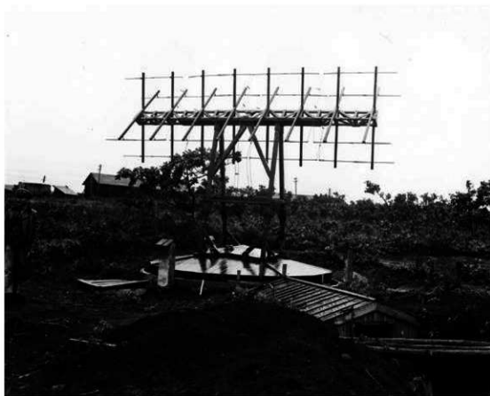
第66図 タチ3号送信機（米国立公文書館）1945年10月8日撮影 工藤洋三氏提供 北海道室蘭市八丁平5丁目、高平（栗山）障地に設置されたもの
