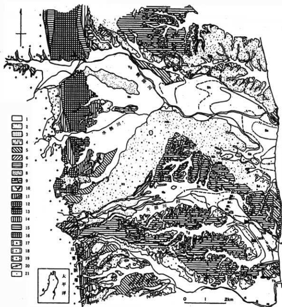
1: "沖積層", 2: 第6段丘構成層, 3: 第5段丘構成層, 4: 第4段丘構成層, 5: 第3段丘構成層, 6: 第2段丘構成層, 7: 第1段丘構成層, 8~11: 電の口層, 8: 同c層(砂岩), 9: 同c層(シルト岩・京塚沢凝灰岩), 10: 同b層, 11: 同a層, 12~19: 基盤岩類, 12: 塚手層, 13: 小山田層, 14: 富沢層, 15: 中の沢層, 16: 柳屋層, 17: 古生層, 18: 花崗岩類, 19: 麻岩, 20: 電の口層上面標高(m), 21: ホーリング地点と孔番, Ah: 畦原, Bb: 馬場, Hi: 雲雀ヶ原, Hm: 原町市街, Ht: 東高松, Ka: 菅浜, Kh: 北原, Kk: 片倉, Mg: 扇形沢, Mm: 米々沢, Nn: 長野, No: 中太田, Om: 大塚, Sd: 幸, Se: 下江井, Sk: 下北高平, So: 下太田, Ss: 下渋谷, Tb: 塚原, Tg: 鶴谷, Tm: 鶴前, Yg: 横上
