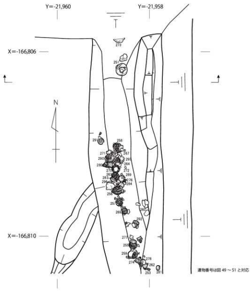
図 29 SD380 平面・断面図 (S = 1/40)
