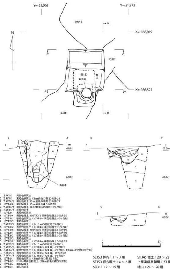
図15 SE153平面・断面図 (S = 1/40)
