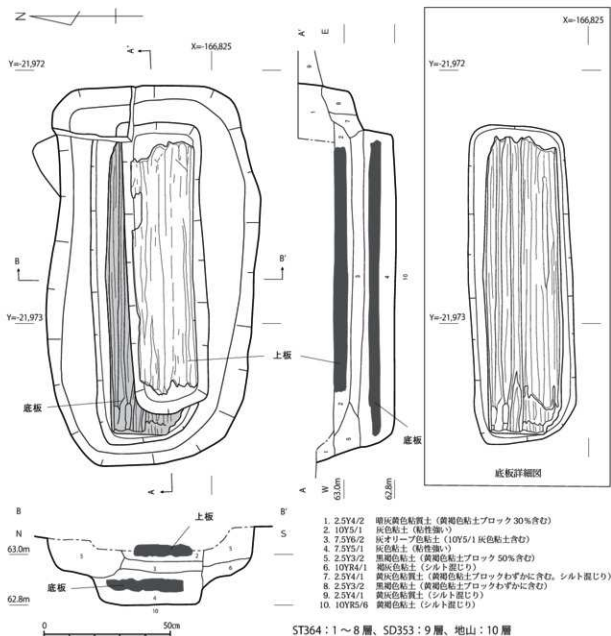
図16 ST364 平面・断面図 (S = 1/15)
