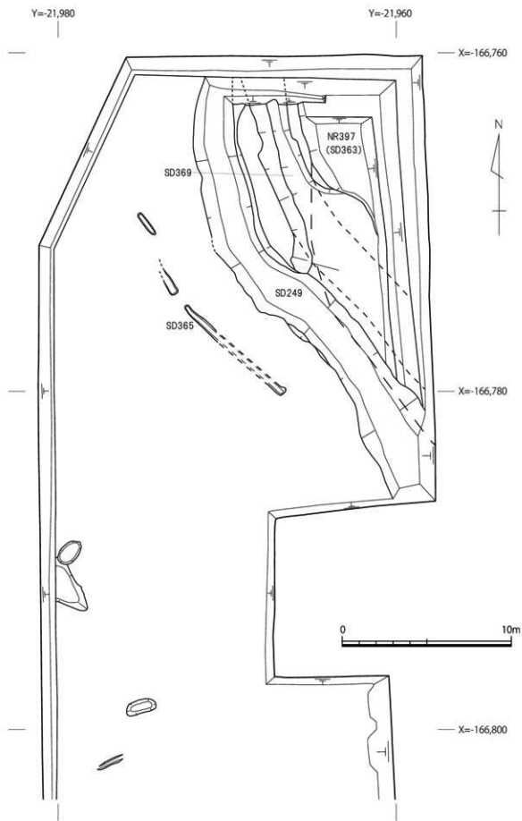
图24 古墳時代初頭遺構平面図① (S = 1/200)
