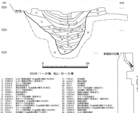
図28 SD249 断面図 (S = 1/40)
