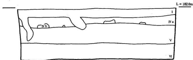
第6図 3トレンチ南壁断面図
