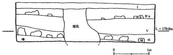
第9図 6 トレンチ北壁断面図
