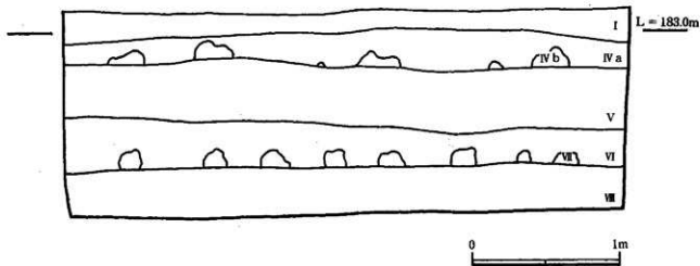
第5図 2 トレンチ南壁断面図
