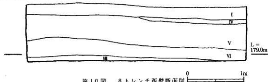
第10図 8 トレンチ西壁断面図
