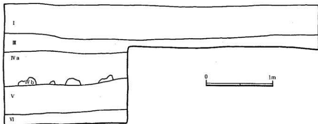
第16図 14トレンチ北壁断面図
