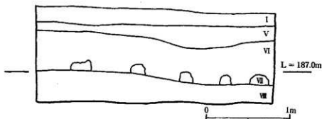
第4図 1 トレンチ北壁断面図
