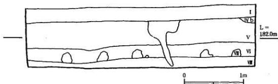
第7図 4トレンチ南壁断面図
