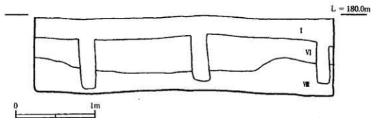
第11図 9 トレンチ西壁断面図
