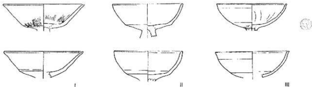
図17 I～IIIの高杯
