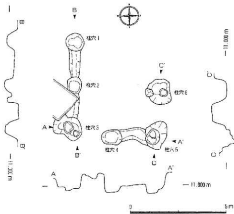
図6 掘立柱建物1 平面図
