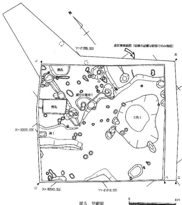
図5 平面図
