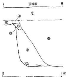
図10 土坑2断面図(水準値記録できず)
