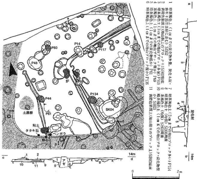
第6図 SB02平・断面図(1:50)
